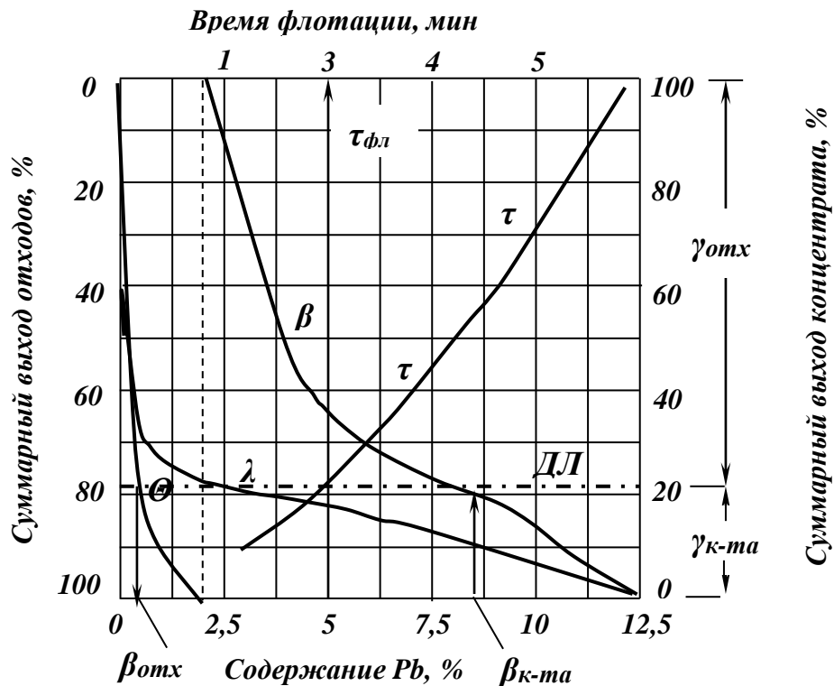
Рис. 3.2 – Кривые флотиремости свинцовой руды
