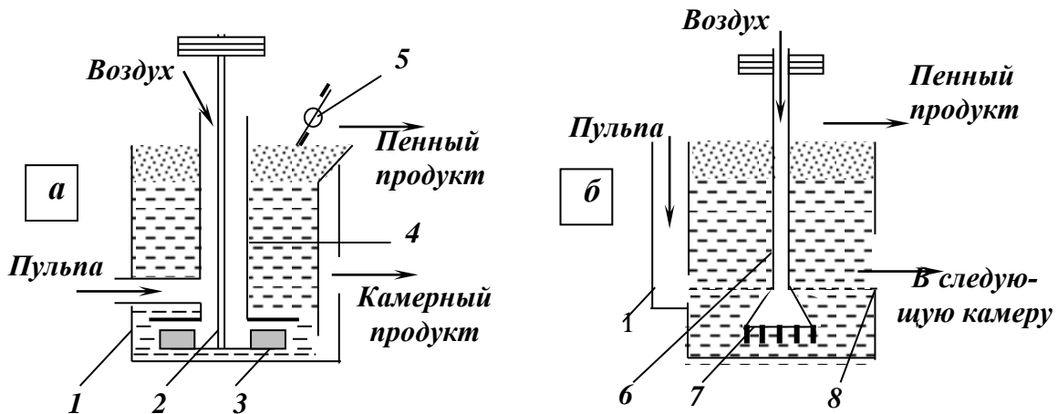
Рис. 6.2 – Схемы флотационных машин
