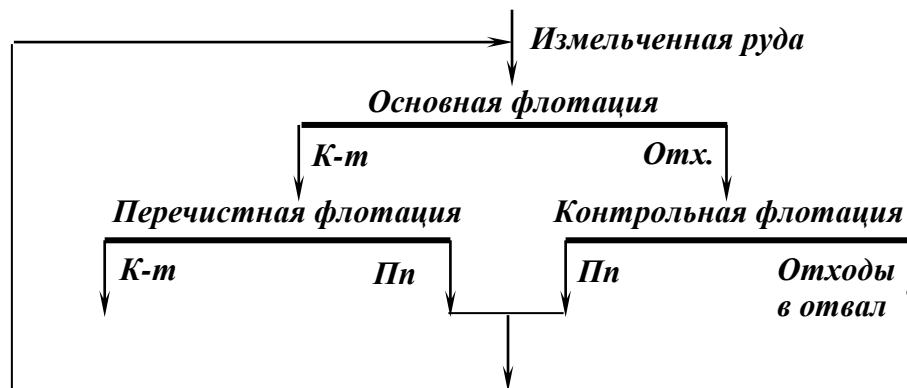
Рис. 6.4 – Операции флотации
