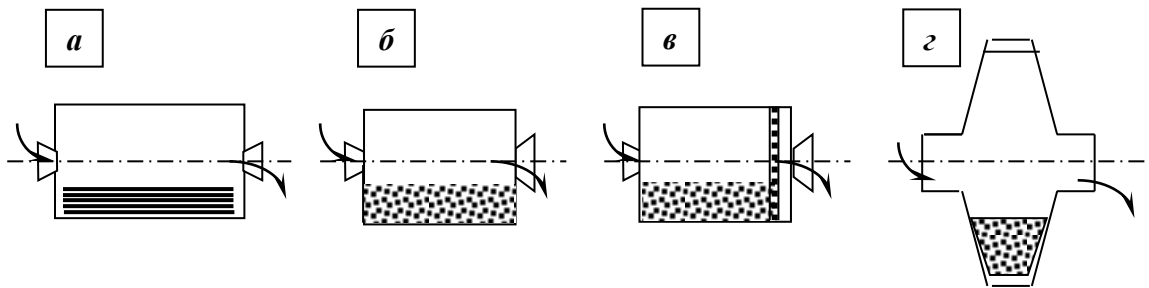
Рис. 5.1 – Барабанные мельницы
