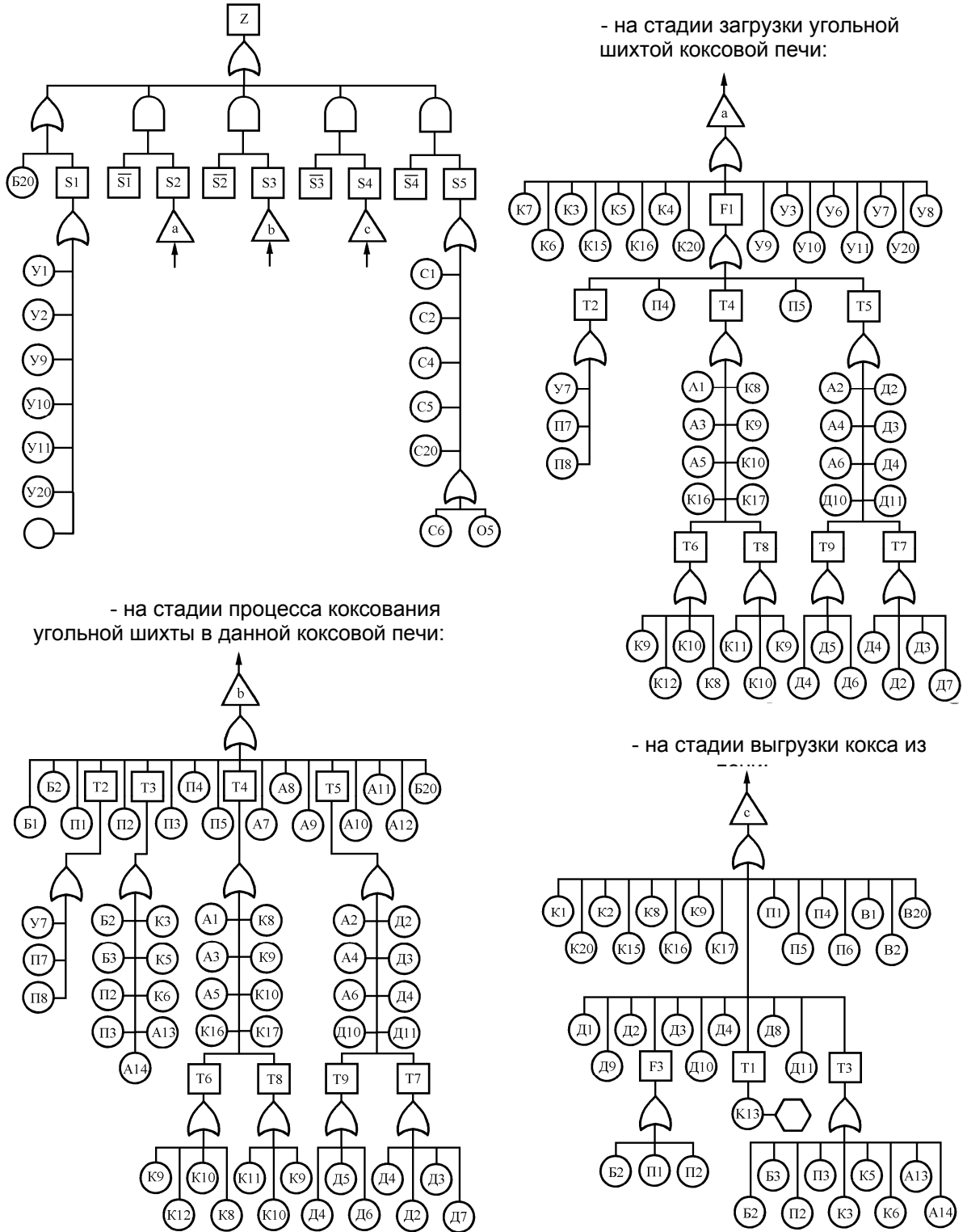
Рис. 1. ДСФ комплекса производства кокса по традиционной технологии
