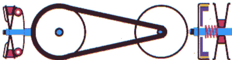
Положения клиновидного ремня в разрезе на ведущем
