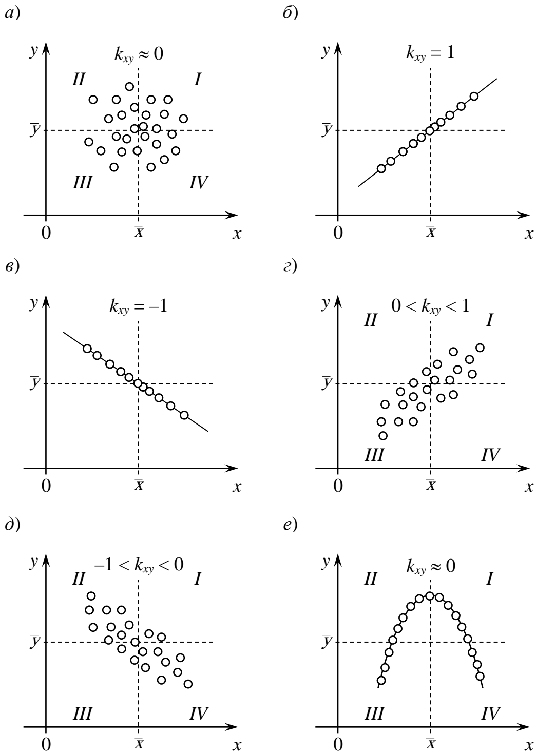
Рисунок 6.1 – Диаграммы рассеяния
