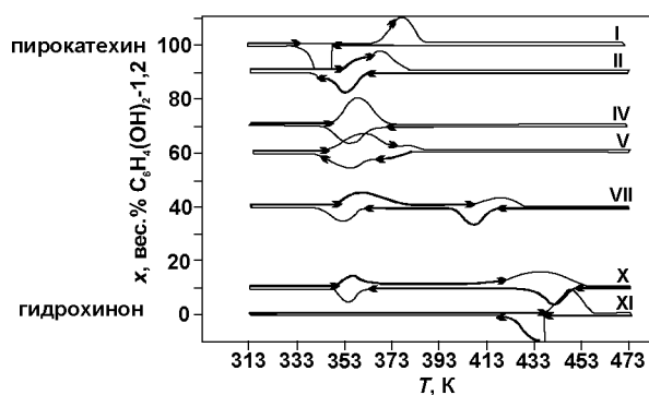
Рис. 2. Экспериментальные ДТА-граммы, характеризующие плавление и кристаллизацию смесей в системе пирокатехин-гидрохинон
