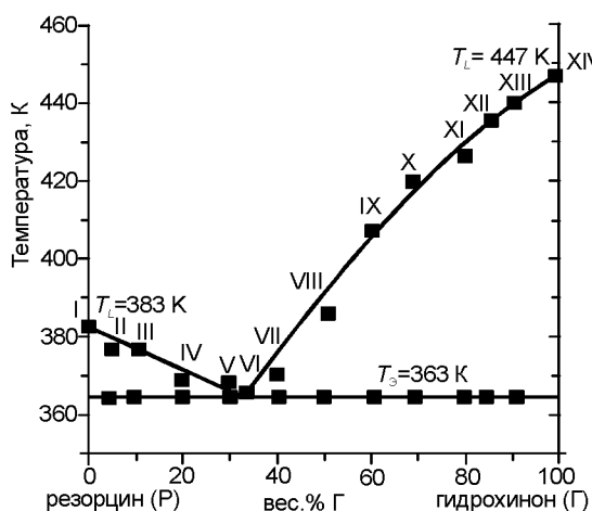
Рис. 4. Диаграмма состояния резорцин – гидрохинон
