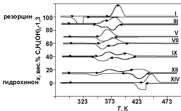
Рис. 3. Экспериментальные ДТА-граммы, характеризующие плавление и кристаллизацию смесей в системе резорцин – гидрохинон
