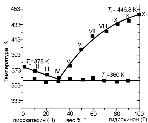
Рис. 5. Диаграмма состояния пирокатехин – гидрохинон
