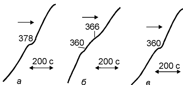
Рис. 1. Термограммы плавления пирокатехина (а), сплава 70% П+30% Г (б) и гидрохинона (в), полученные методом ТА. Температуры даны в градусах Кельвина.
