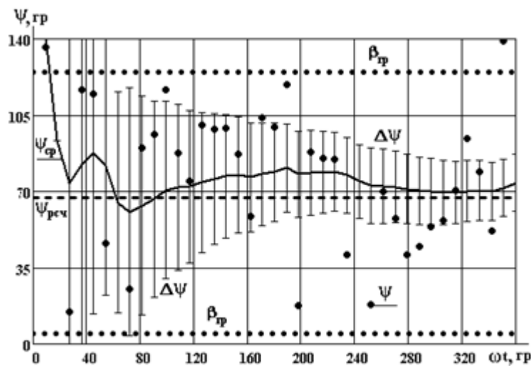
Рисунок 6 - Работа БПР при R_h = 14 кОм: \psi , \psi_{cp} , \psi_{рсч} – текущее, среднее и расчетное значения аргумента ПН; \Delta\psi – доверительный интервал среднего; \beta_{гр} - границы ОФИ
