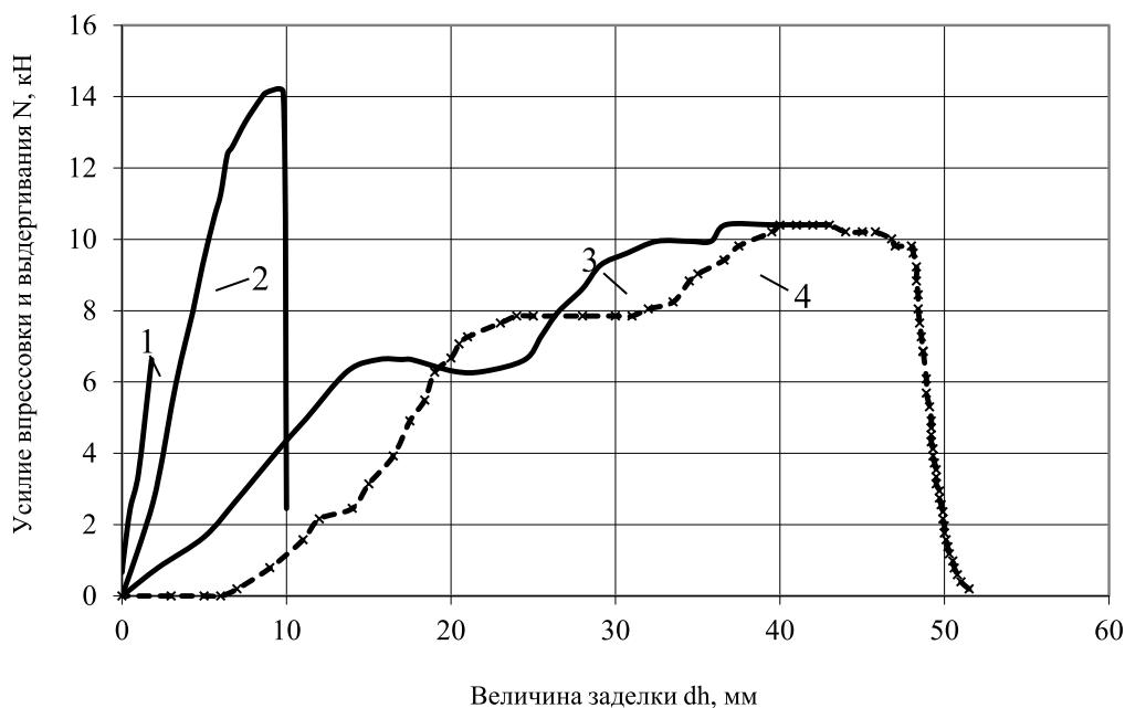
Рис. 1 – Зависимость усилия впresseвки и выдергивания анкера от величины заделки: 1, 2, 3 – зависимость усилия впresseвки от глубины заделки при превышении диаметра анкера над диаметром шпура соответственно на 3,8; 2,5 и 1,3%; 4 - зависимость усилия выдергивания от глубины заделки
