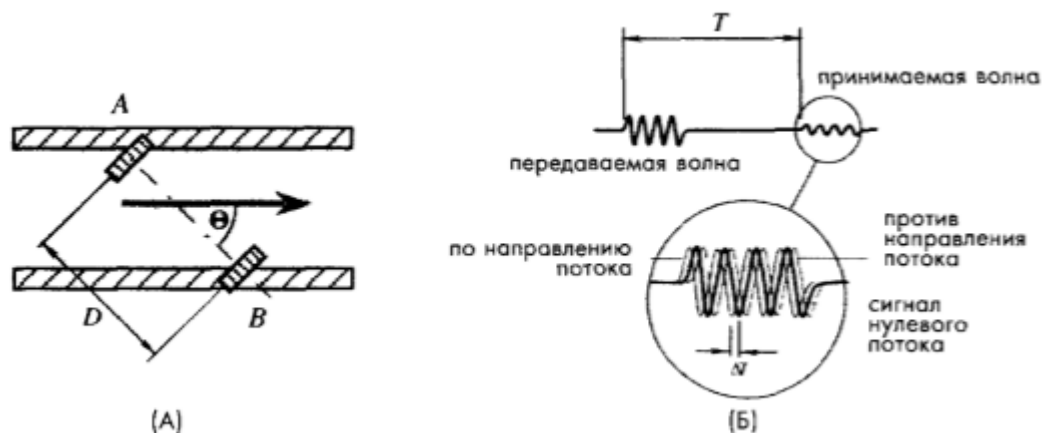
Рисунок 1 – Ультразвуковой расходомер. А – положение приемно-передающих кристаллов в потоке среды, Б – форма звуковых волн
