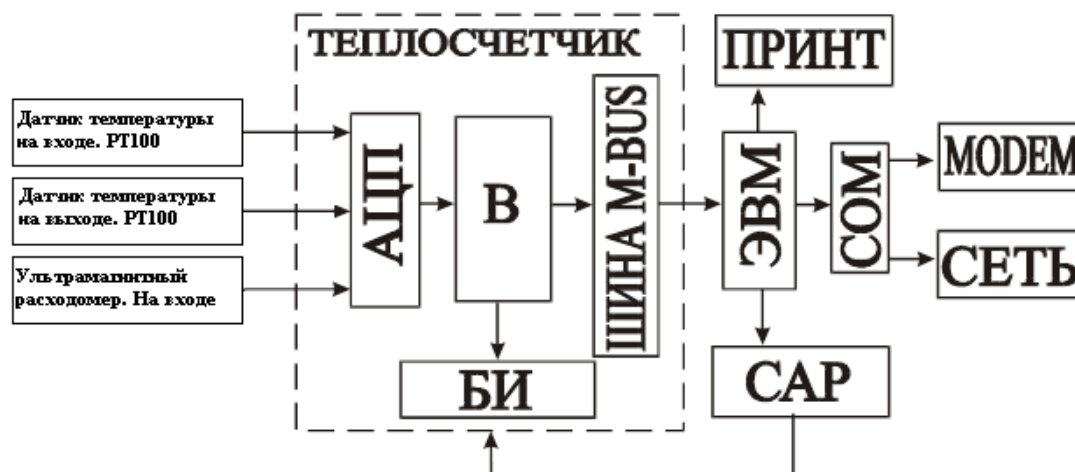
Рисунок 3 – Структурная схема теплосчетчика
