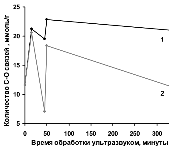
Рис. 3. Зависимость содержания связей С-О в грубой (1) и мелкой фракциях (2) от времени обработки ультразвуком
