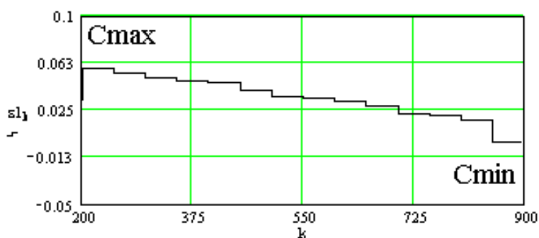
Рисунок 7 – Распределение погрешности измерения по градуировочным уровням (Cmax и Cmin – максимальное и минимальное значения измеряемой концентрации)
