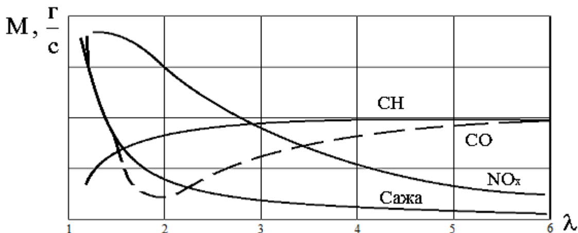
Рисунок 1 – Влияние коэффициента избытка воздуха \lambda на выбросы автотранспорта M
