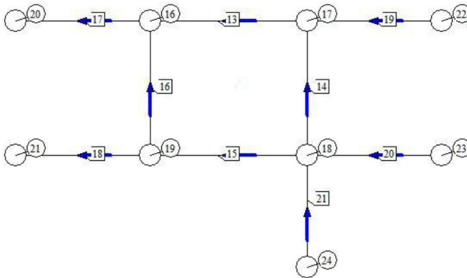
Рис. 5.9 – Схема соединений вентиляционного контура
