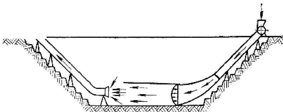
Рис. 24.9 – Схема нагнетательно-всасывающей вентиляции вентиляторными установками с применением трубопроводов
