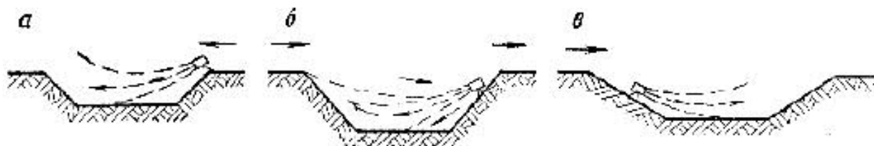
Рис. 24.10 – Схемы вентиляции карьеров вентиляторной установкой
