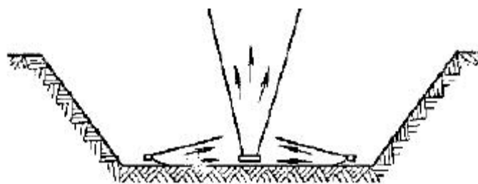
Рис. 24.16 – Комбинированная схема вентиляции карьера вертикальной и горизонтальными струями
