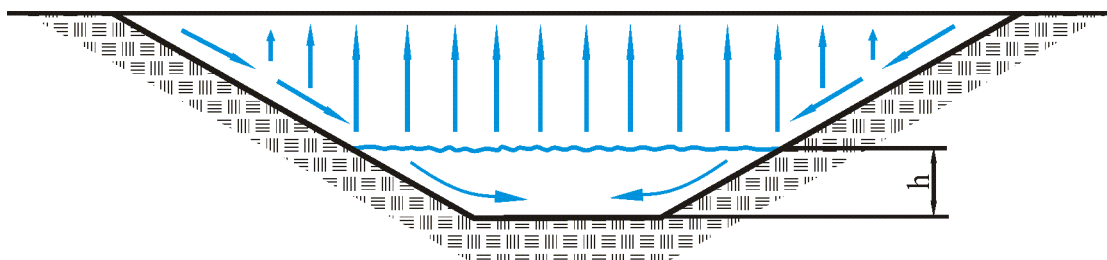
Рис. 23.6 – Движение воздуха в карьере при инверсионной схеме
