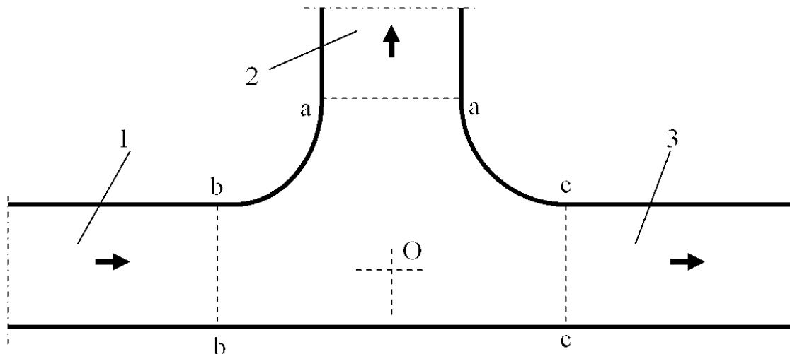
Рис. 21.1 – Место соединения (сопряжения) трех выработок или частей выработок
