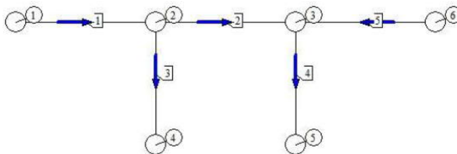
Рис. 5.8 – Схема вентиляционного соединения
