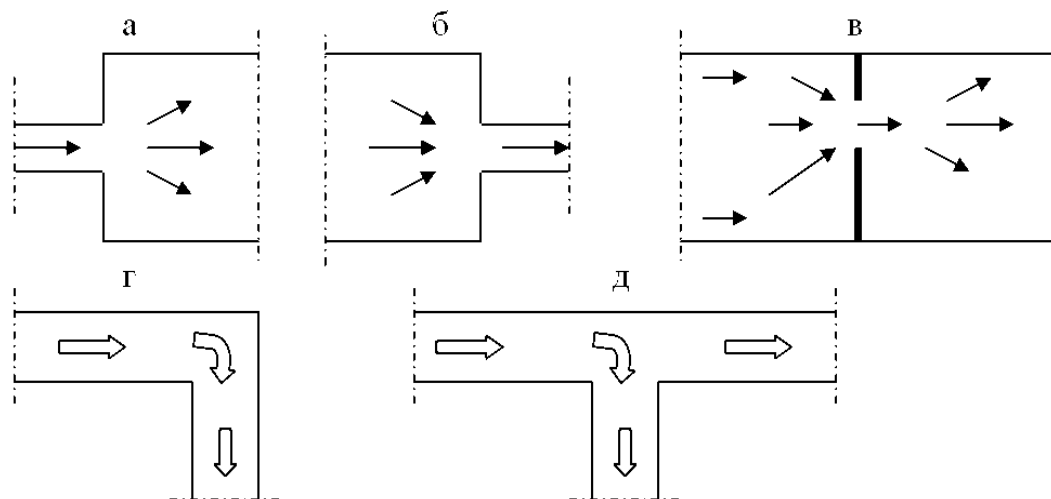
Рис. 4.1 – Местные сопротивления в горных выработках
