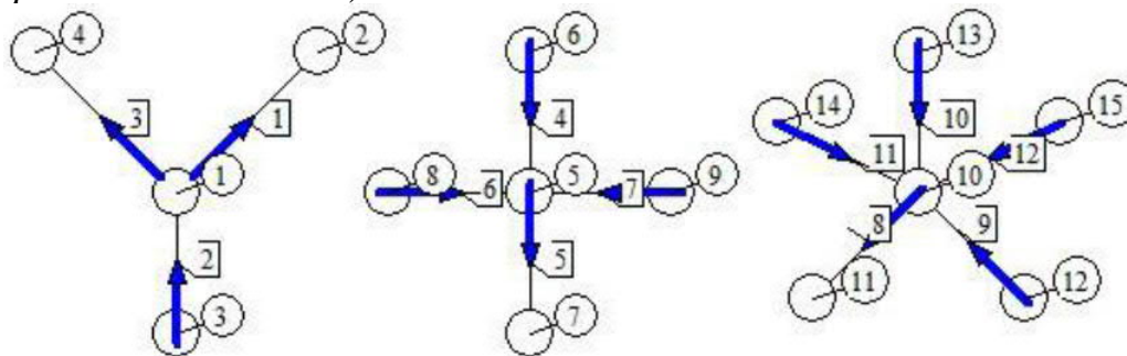
Рис. 5.6 – Схемы вентиляционных соединений типа «звезда»
