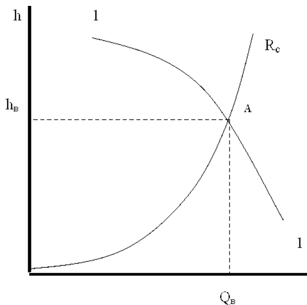
Рис. 7.3 – Определение режима работы вентилятора
