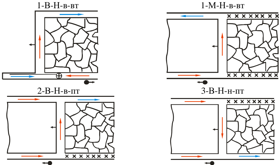
Рис. 13.1 – Варианты схем проветривания выемочных участков
