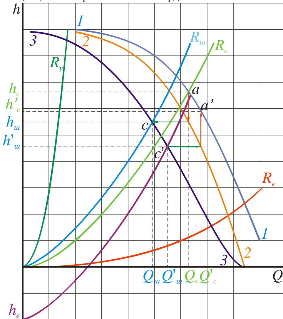
Рис. 6.3 – Определение режима проветривания шахты
