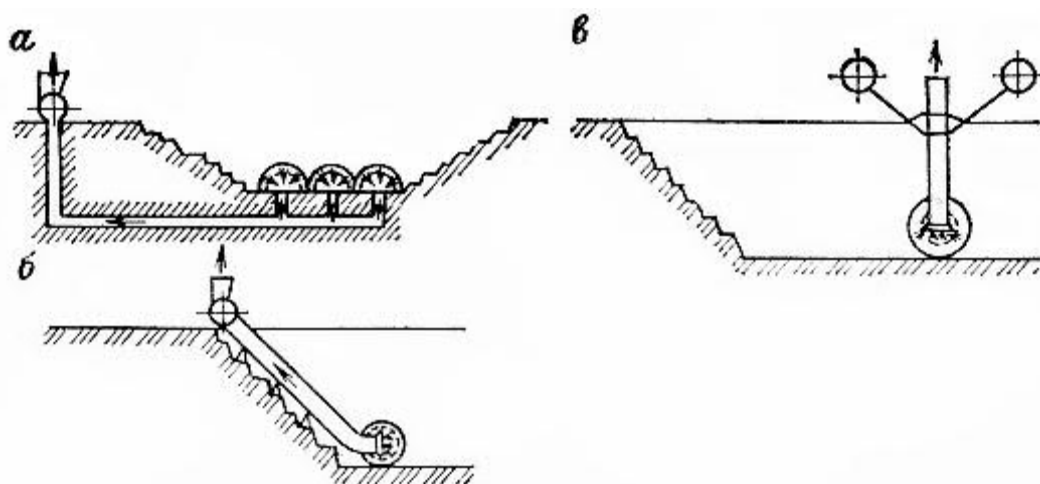
Рис. 24.4 – Варианты всасывающего проветривания карьера:
