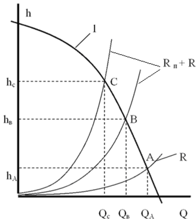
Рис. 20.2 – Определение параметров приведенной характеристики
