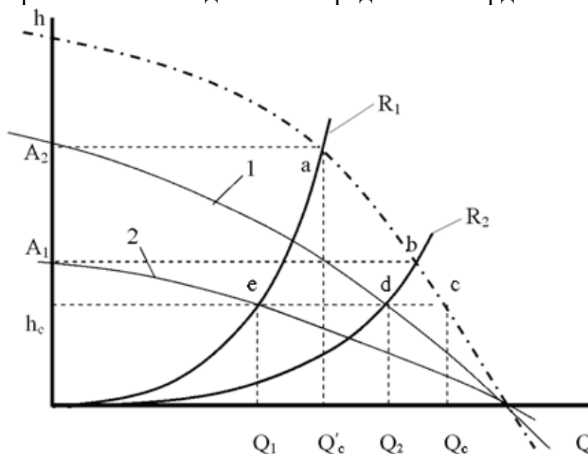
Рис. 20.1 – Формирование режима проветривания параллельного соединения
