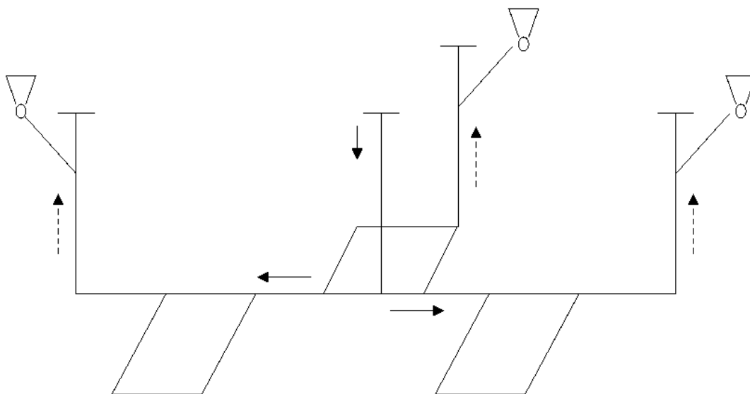
Рис. 15.4 – Комбинированная схема вентиляции шахты
