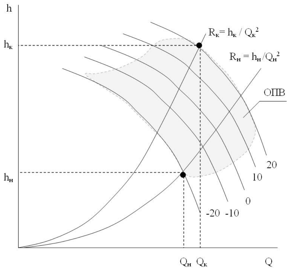
Рис. 16.1 – Область промышленного использования вентилятора
