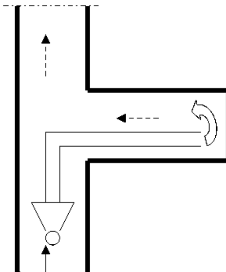
Рис. 14.2 – Схема нагнетательного проветривания тупиковой выработки
