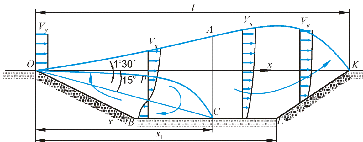
Рис. 23.3 – Рециркуляционно-прямоточная схема проветривания карьера
