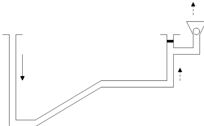
Рис. 15.2 – Центрально отнесенная схема вентиляции шахты
