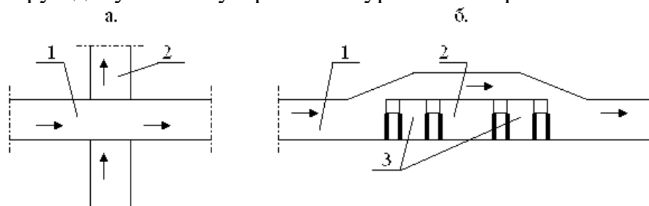
Рис. 8.3 – Упрощенная схема движения воздуха по кроссингу а – схема пересечения выработок; б – схема кроссинга
