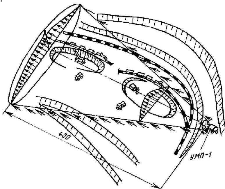
Рис. 24.5 – Схема вентиляции и гидрообеспыливания застойной зоны одиночной струей
