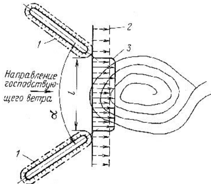
Рис. 24.2 – Схема воздухозабора: 1 – отвалы; 2 и 3 – эпюры скорости ветрового потока над карьером соответственно при отсутствии и наличии воздухозабора
