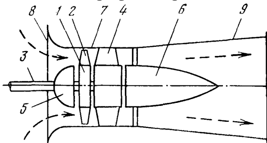
Рис. 7.1 – Схема осевого вентилятора
