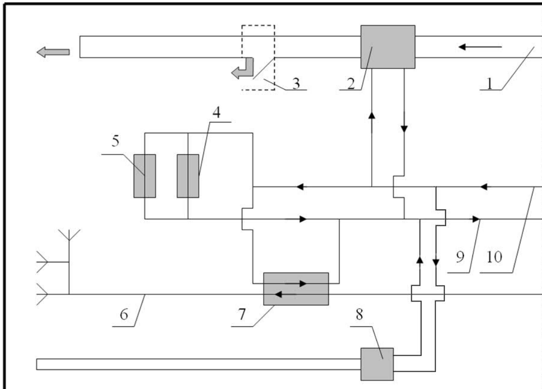
Рис. 12.2 – Схема кондиционирования воздуха в призабойной зоне тупиковой выработки с комбайновой проходкой
