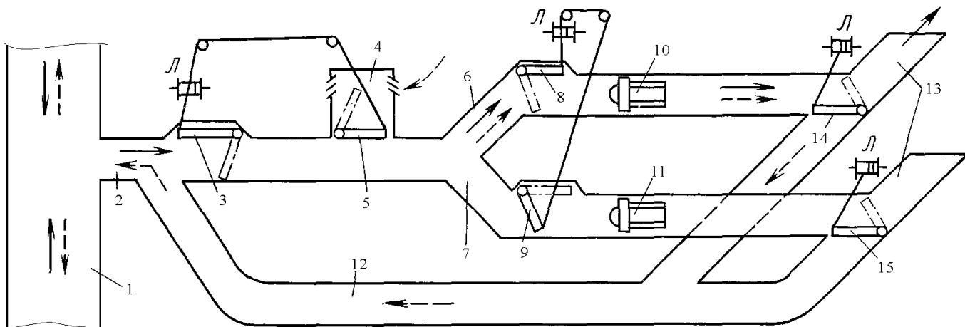
Рис. 8.1 – Схема каналов вентиляторной установки:
