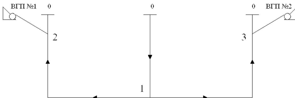
Рис. 9.2 – Схема проветривания шахты с двумя фланговыми вентиляторами
