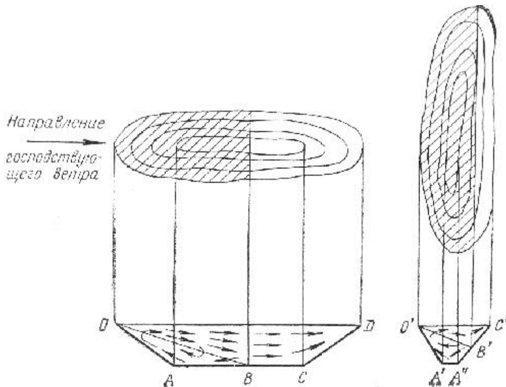
Рис. 24.1 – Ориентация карьера в плане относительно направления господствующего ветра
