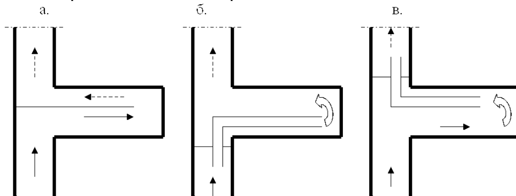
Рис. 14.1 – Схемы проветривания тупиковой выработки с помощью перегородки (а) и жесткой вентиляционной трубы (б, в)
