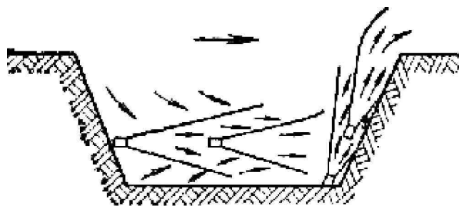
Рис. 24.13 – Схема вентиляции глубокого карьера каскадными восходящими струями
