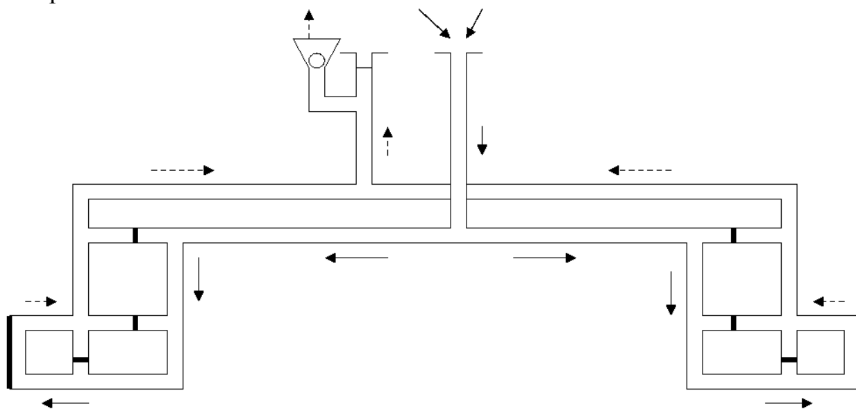
Рис. 15.1 – Центрально-сдвоенная схема вентиляции шахты
