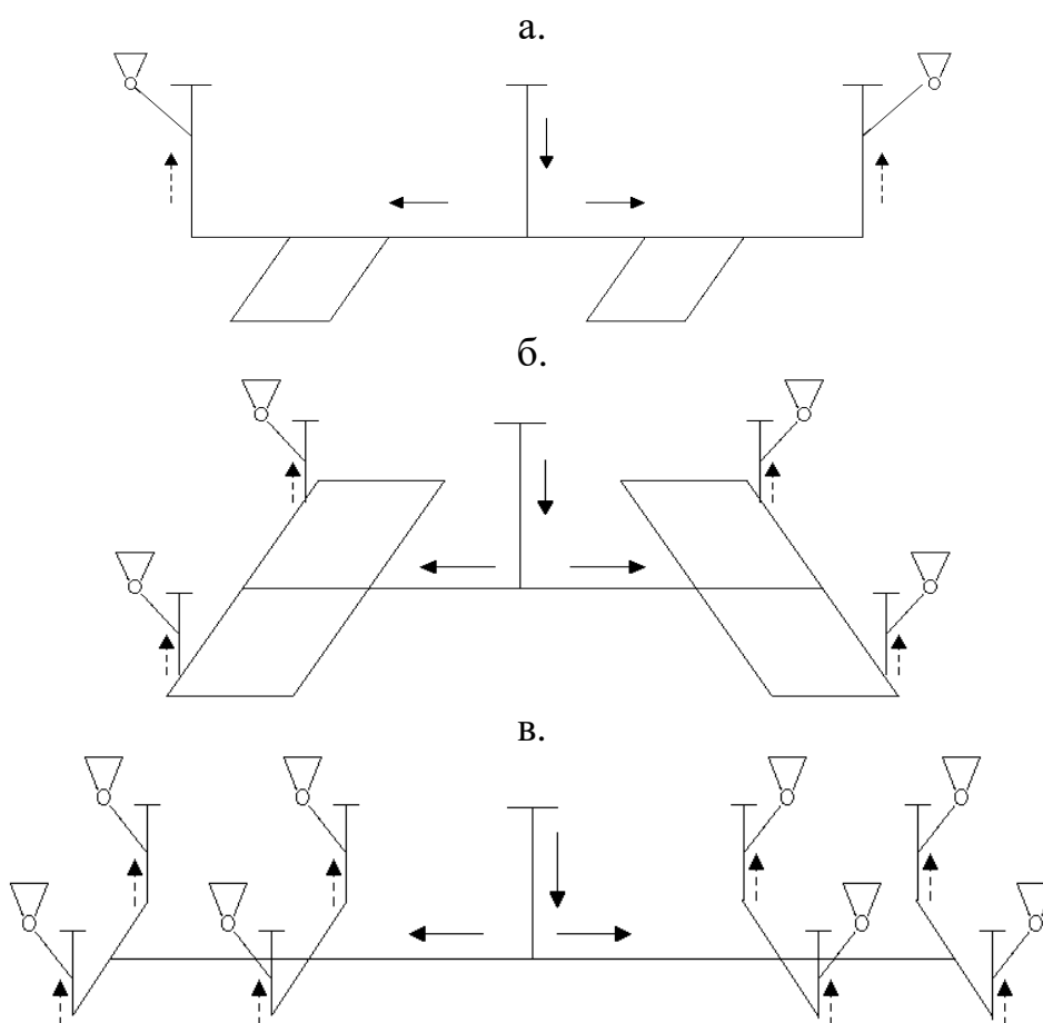
Рис. 15.3 – Фланговые схемы вентиляции шахт: а – крыльевая; б – групповая; в – участковая
