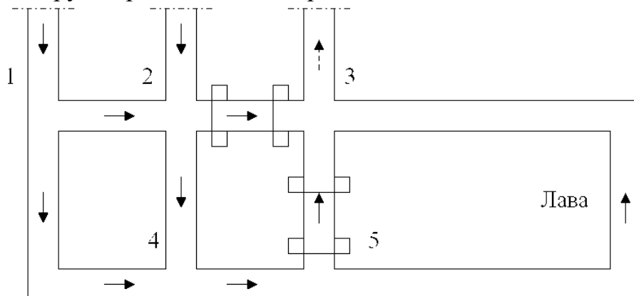
Рис. 17.3 – Схема вентиляции выемочного участка
