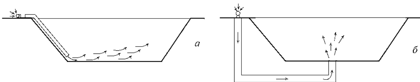
Рис. 24.3 – Схема проветривания карьера нагнетательным способом: а – с применением труб и б – с использованием выработок
