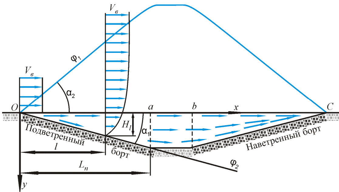
Рис. 23.1 – Прямоточная схема проветривания карьера
