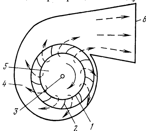
Рис. 7.2 – Схема центробежного вентилятора
