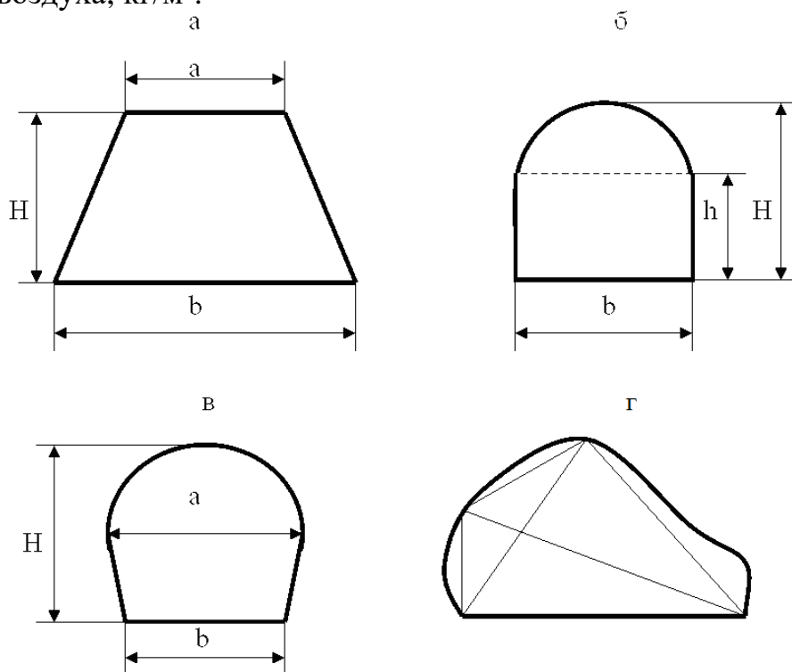
Рис. 19.2 – Схемы поперечных сечений горных выработок
