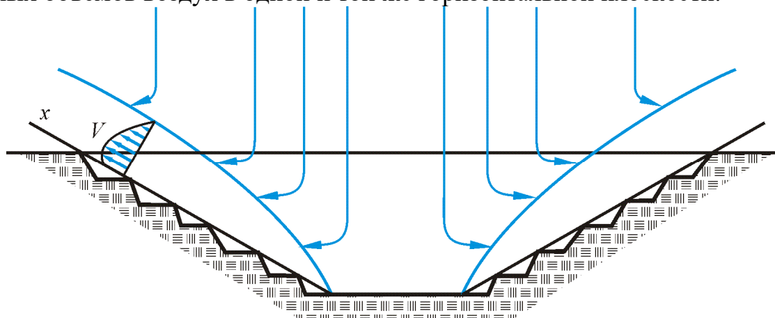
Рис. 23.5 – Конвективная схема проветривания карьера
