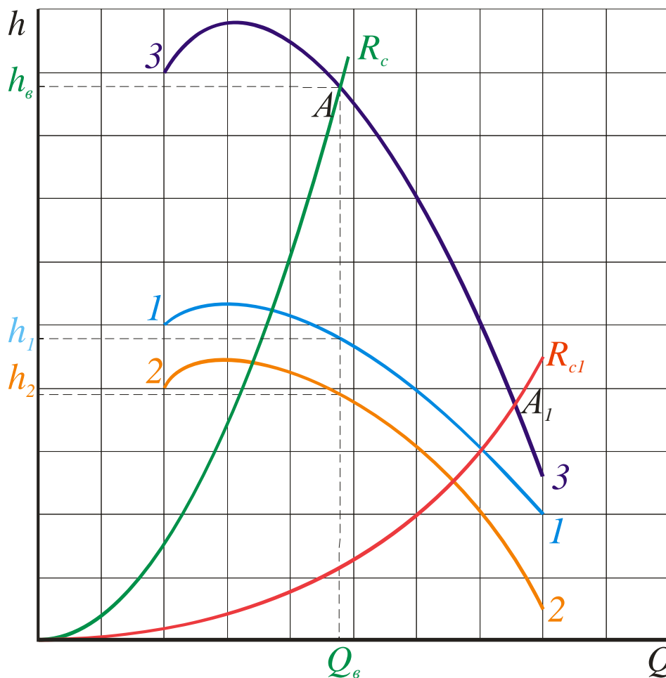
Рис. 7.4 – Характеристика последовательно работающих вентиляторов
