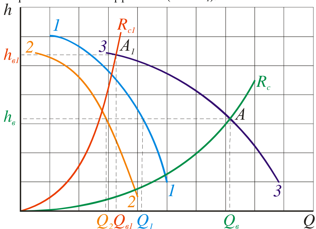
Рис. 7.5 – Характеристика параллельно работающих вентиляторов
