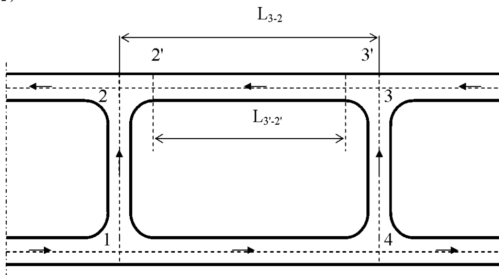
Рис. 21.2 – Схема соединения горных выработок в вентиляционном контуре
