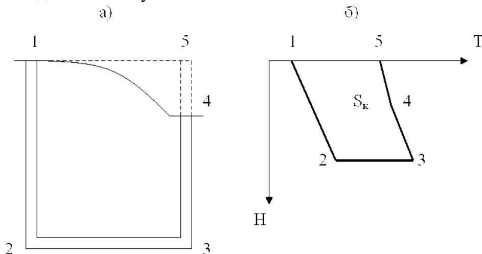
Рис. 6.1 – Схема горных выработок с естественной тягой
