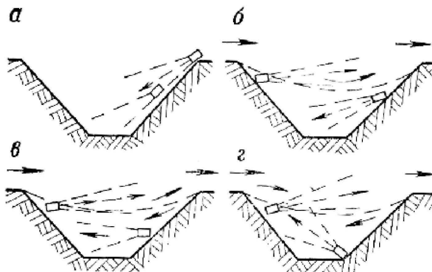
Рис. 24.14 – Схемы вентиляции глубокого карьера двумя последовательно работающими вентиляторными установками
