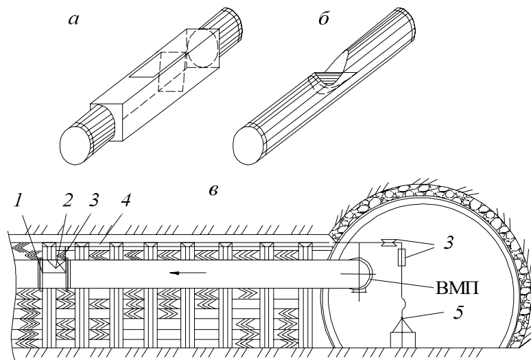
Рис. 14.5 – Устройство для разгазирования тупиковых горных выработок: а, б – схемы устройства; в – схема установки; 1 – патрубок; 2 – клапан; 3 – ролики; 4 – трос; 5 – ручная (электрическая) лебедка
