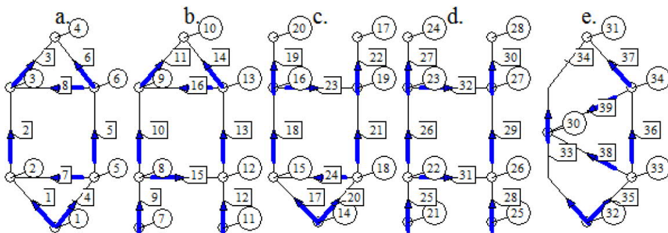
Рис. 17.2 – Схемы сложных вентиляционных соединений с двумя диагоналями
