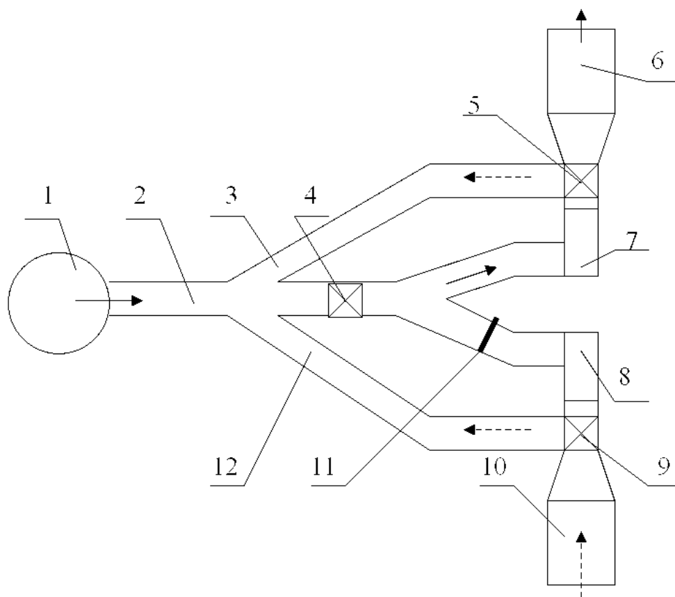
Рис. 8.2 – Схема вентиляторной установки с центробежными вентиляторами:
