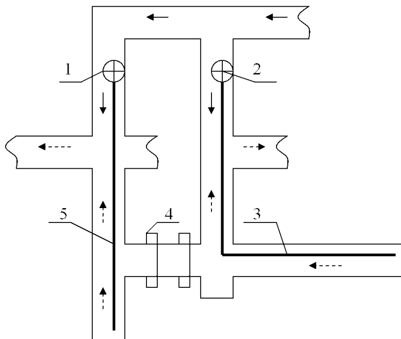
Рис. 14.4 – Схема проветривания тупиковых забоев 1, 2 – ВМП; 3, 5 – трубопроводы; 4 – вентиляционные двери
