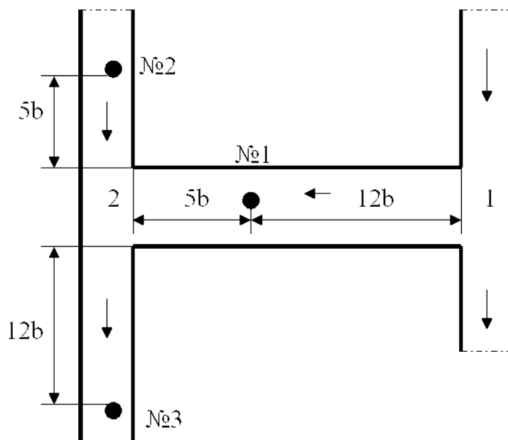
Рис. 19.1 – Схема измерения скорости воздуха в выработках
