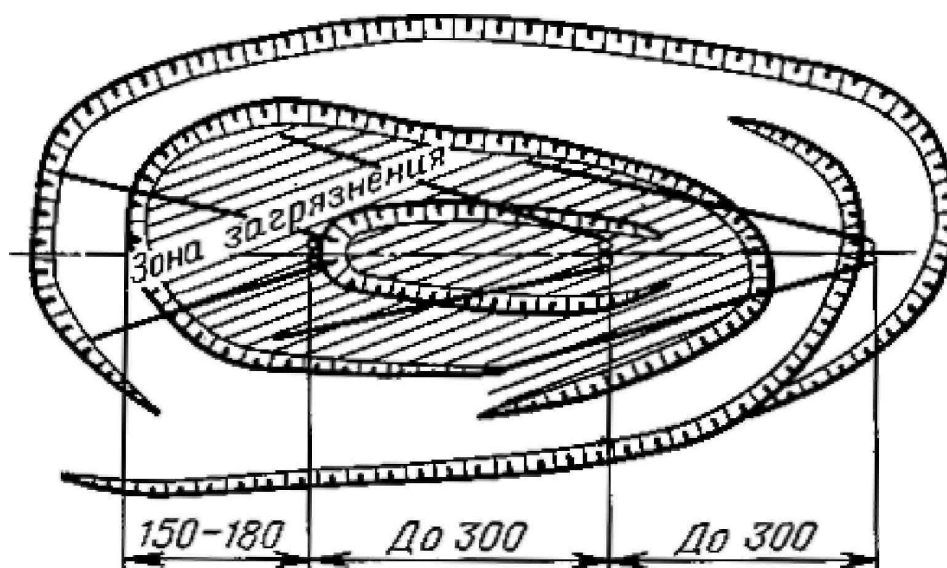
Рис. 24.7 – Схема вентиляции застойной зоны карьера с помощью каскадно расположенных установок
