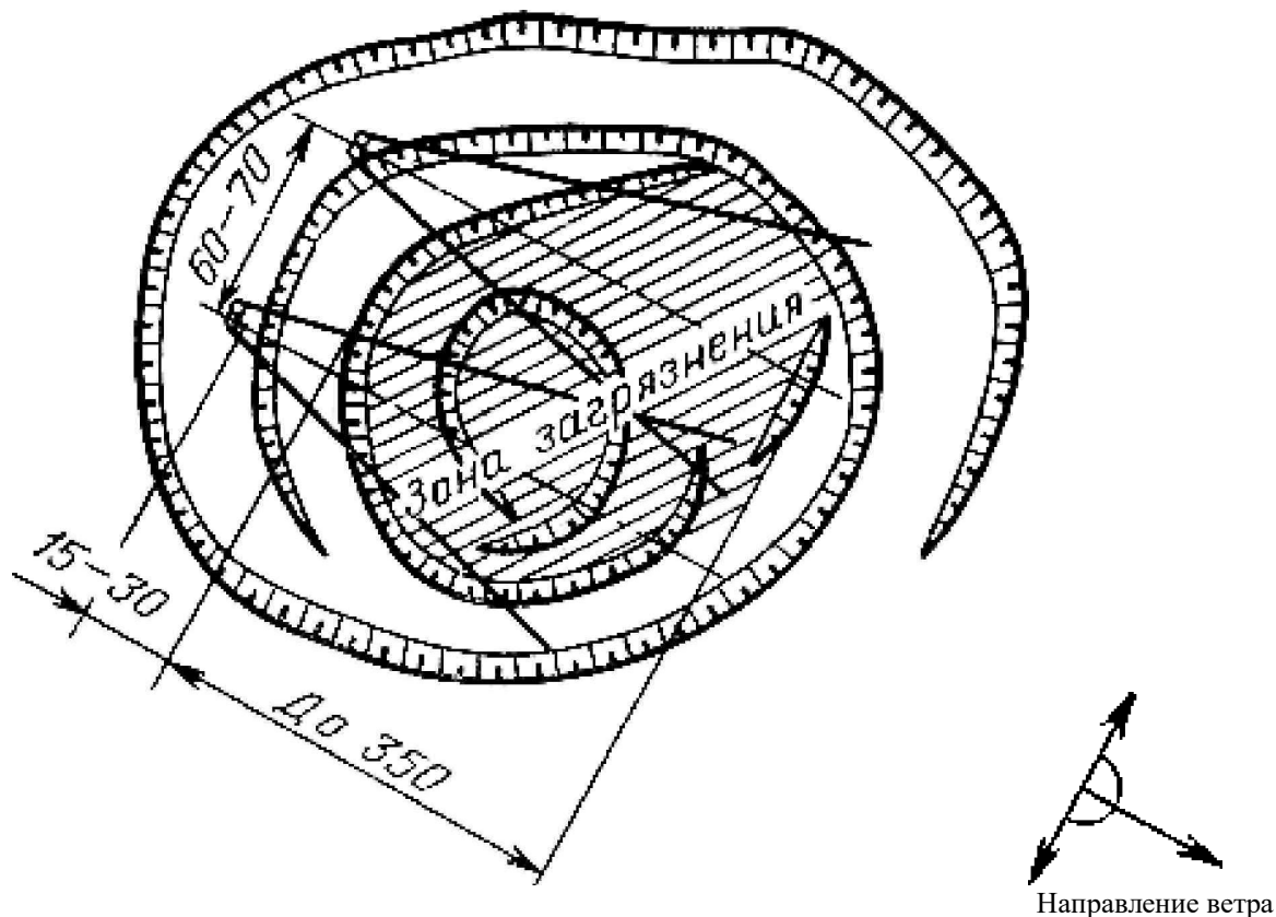
Рис. 24.6 – Схема вентиляции застойной зоны карьера параллельными струями
