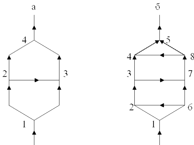
Рис. 17.1 – Схемы диагональных соединений: а – простого, б – сложного
