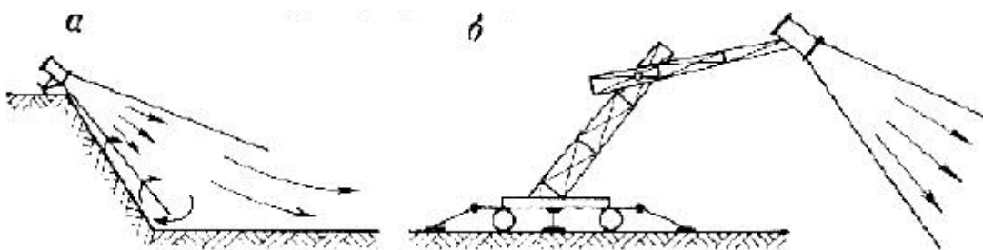
Рис 24.8 – Схемы расположения вентиляторов местного проветривания: а – на верхнем уступе; б – на специальной ферме
