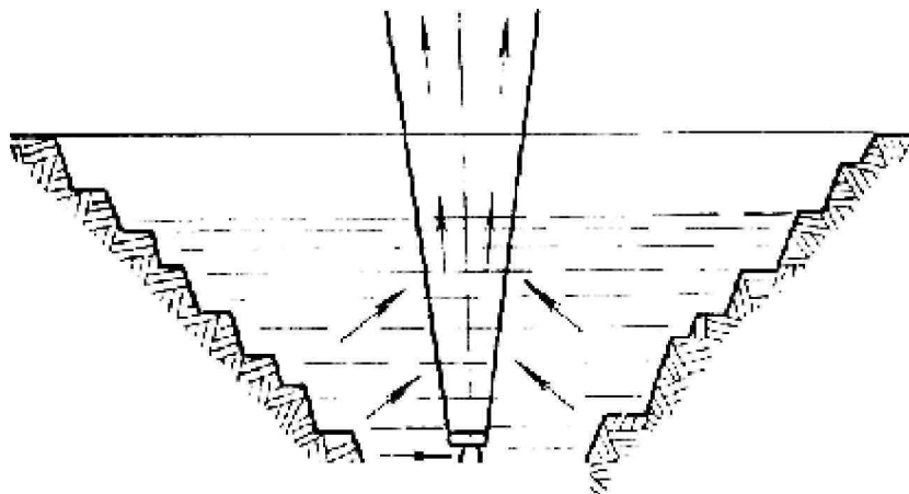
Рис. 24.11 – Схема вентиляции карьера вентиляторной установкой, расположенной на дне карьера и создающей вертикальную струю
