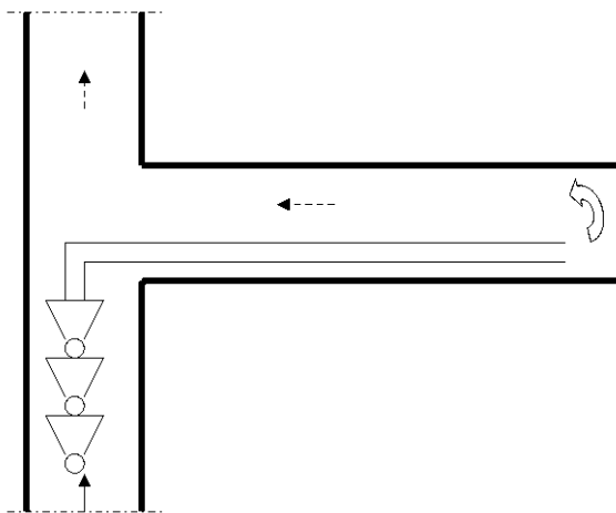
Рис. 14.3 – Схема каскадной установки ВМП
