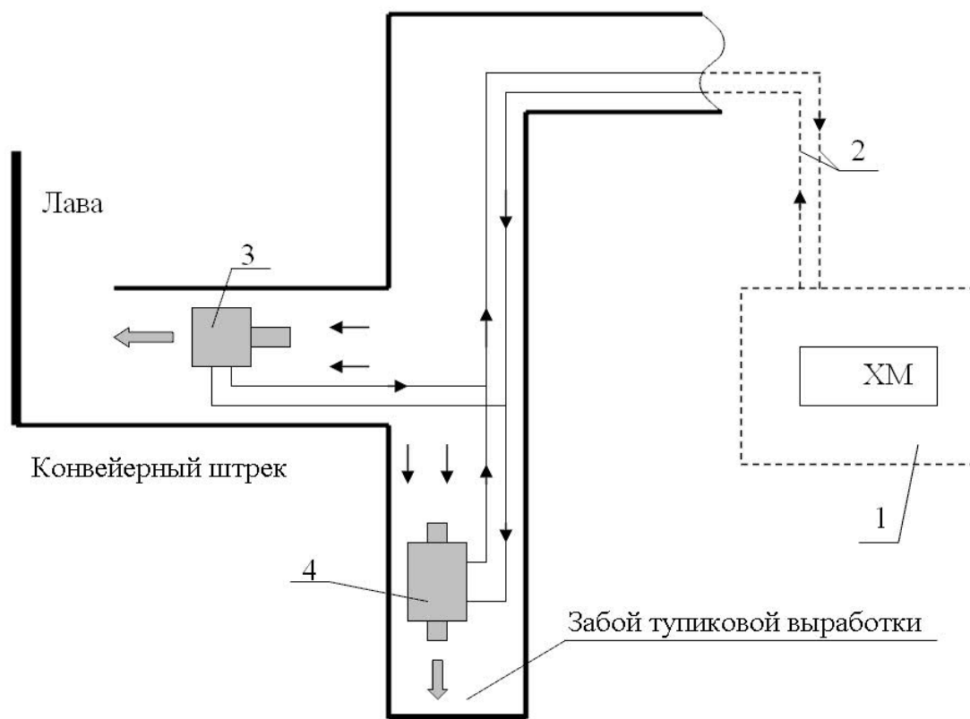
Рис. 12.1 – Схема системы подземного кондиционирования воздуха: 1 – холодильная машина; 2 – трубопроводы с хладоносителем; 3 – штрековый воздухоохладитель; 4 – тупиковый воздухоохладитель
