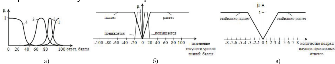
Рисунок 5 – Функции принадлежности нечетким множествам: а) 1- правильный, 2- близкий к правильному, 3 – неточный, 4 – ошибочный; б) падает, понижается, повышается, растет; в) стабильно растет и стабильно падает.
