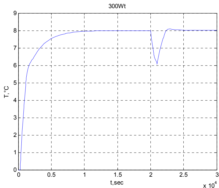
Рис. 8 – График изменения температуры при использовании второго способа регулирования
