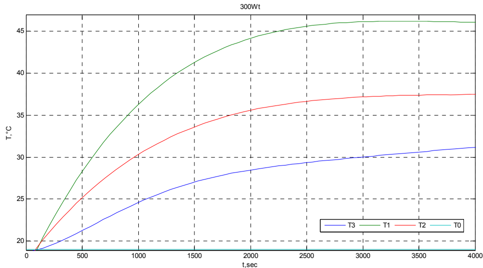
Рис.2 – Аппроксимированные экспериментальные графики температуры для мощности нагревателя 330Вт
