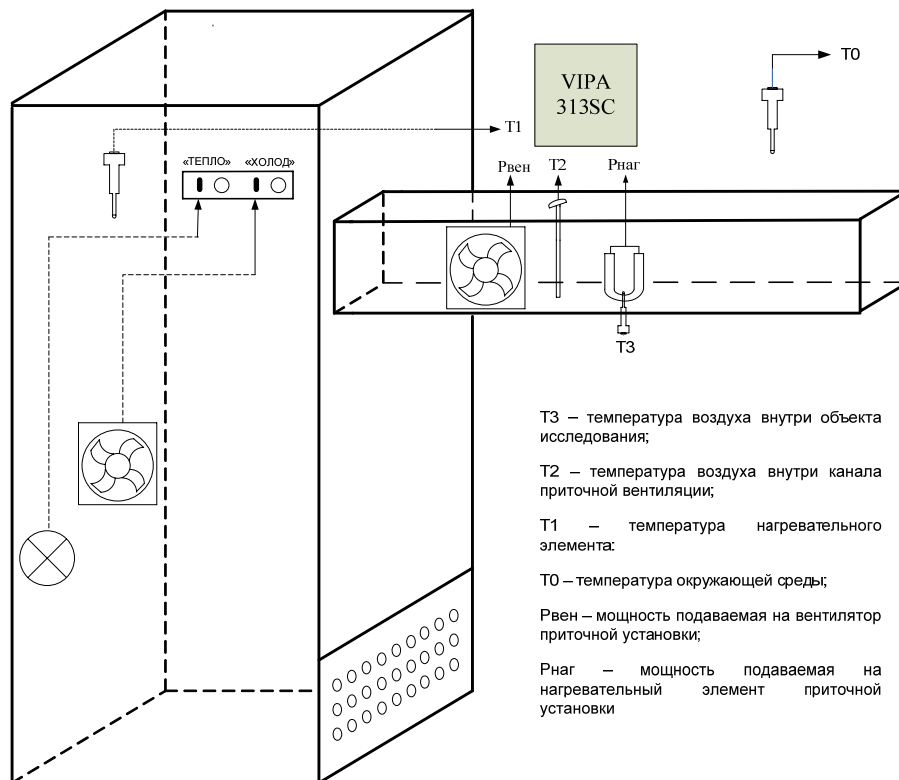
Рис.1 – Структурная схема работы системы приточной вентиляции
