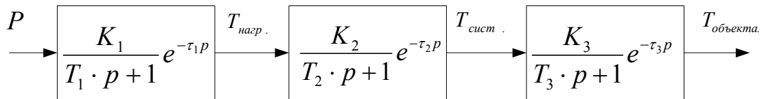
Рис.3 – Структурная схема системы вентиляции
