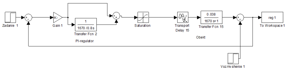
Рис.6 – Модель системы приточной вентиляции с ПИ-регулятором
