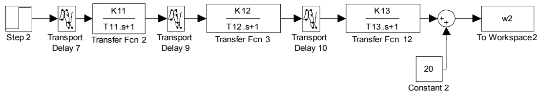
Рис.4 – Модель системы, состоящая из трех звеньев в Simulink для мощности нагревателя 330Вт
