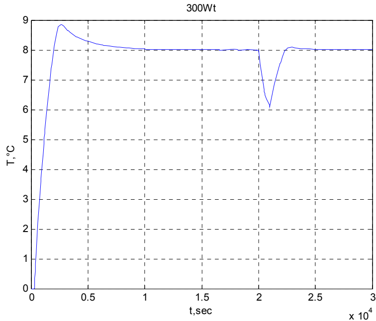
Рис. 7 – График изменения температуры при использовании первого способа регулирования
