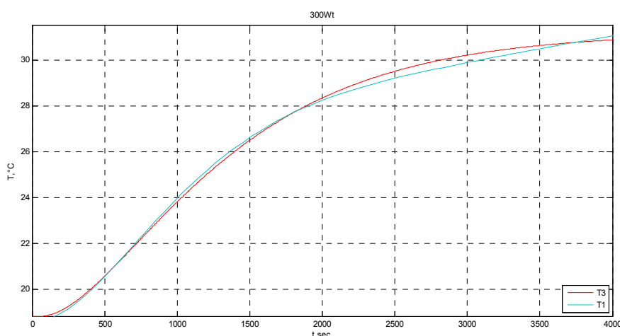
Рис.5 – Графики изменения температуры для мощности нагревательного элемента 330 Вт: T1 – экспериментальный; T3 – полученный в результате моделирования
