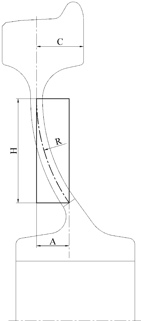
Рисунок 2 – Однорядусный диск колёса (радиус оси диска определён с учётом прогиба цепной линии)
