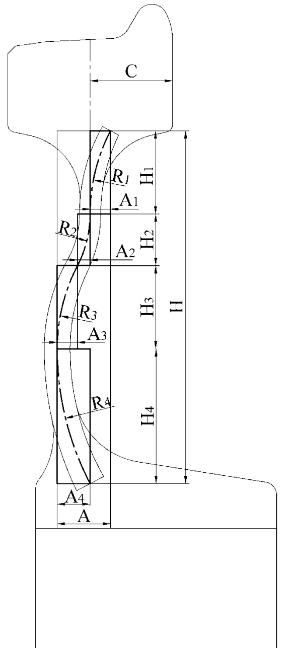
Рисунок 7 – Четырехрадиусный диск колеса (учтены следующие соотношения:
