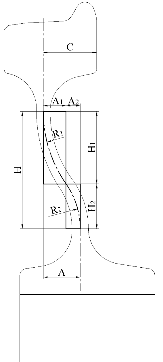
Рисунок 3 – Двухрадиусный диск колёса (учтены следующие соотношения.
