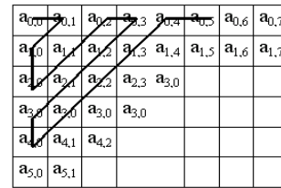
Рисунок 2. – Зигзаг-сканирование
