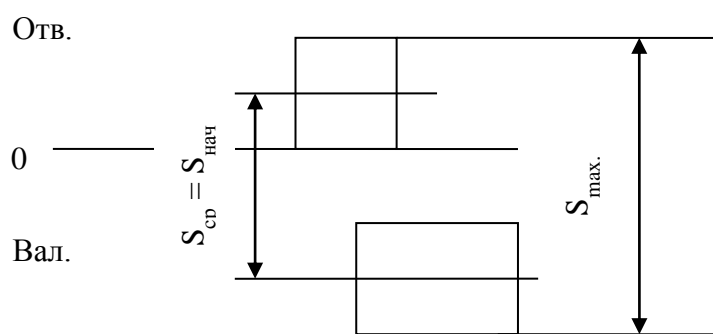
Поле допуска посадки: отверстие-вал
