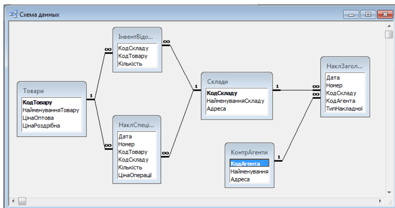
Рисунок 6.1 – Схема даних
