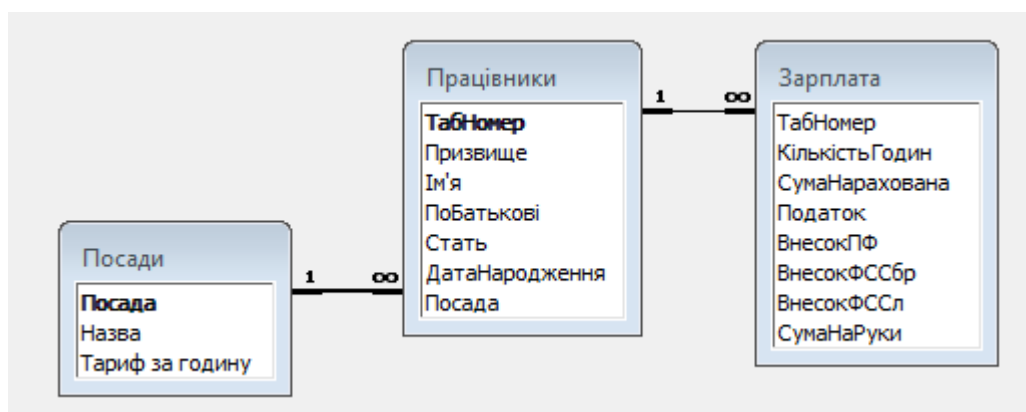
Рисунок 5.1 – Схема даних
