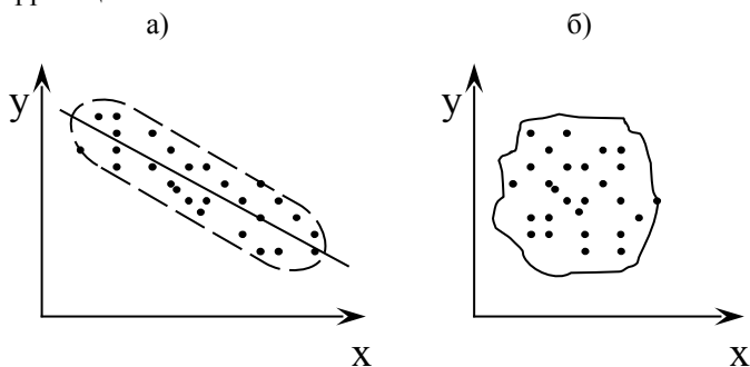
Рисунок 4.8 – Корреляционное поле
