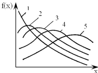
Рисунок 3.11 – Общий вид кривых гамма-распределения
