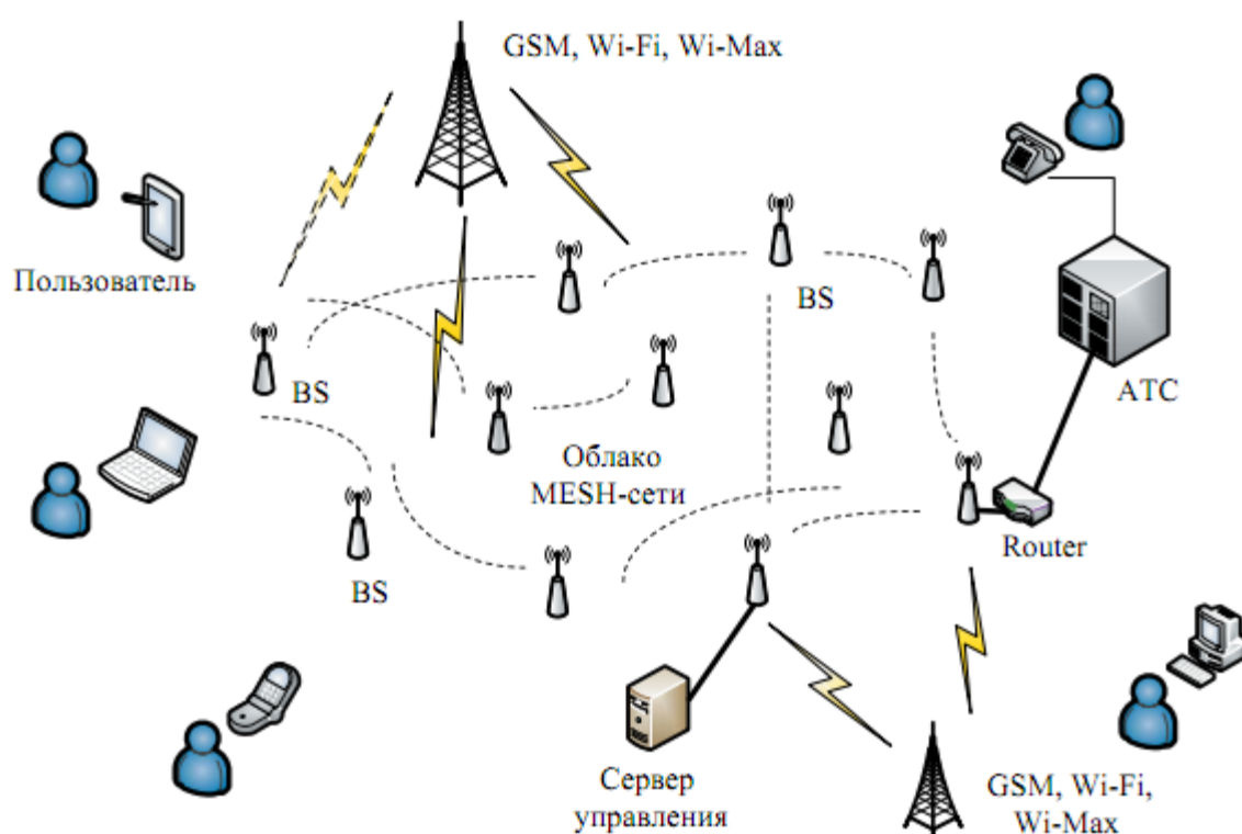
Рисунок 1. Топология Mesh-сети
