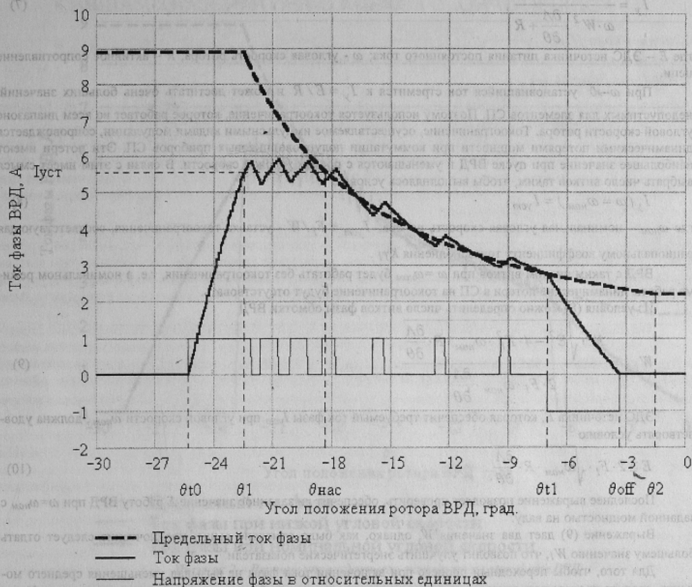
Рисунок 1 – Ток фазы ВРД
