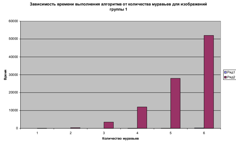
Рис. 5 - Зависимость времени выполнения алгоритма от количества муравьев для изображений группы 1
