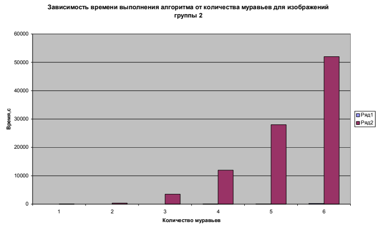
Рис. 6 - Зависимость времени выполнения алгоритма от количества муравьев для изображений группы 2
