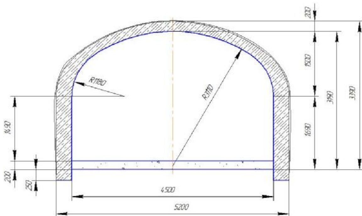
Рисунок 2. Бетонне кріплення
