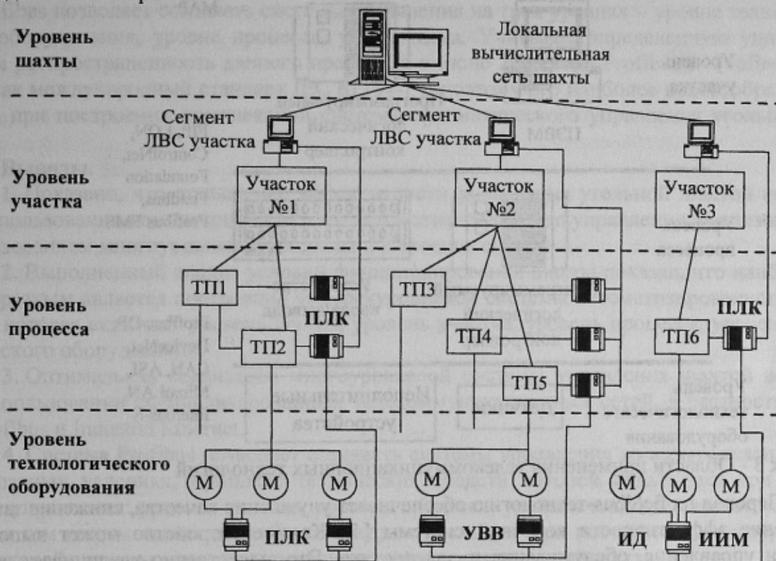
Рисунок 2 – Структура комплексной автоматизированной системы управления шахтой.
