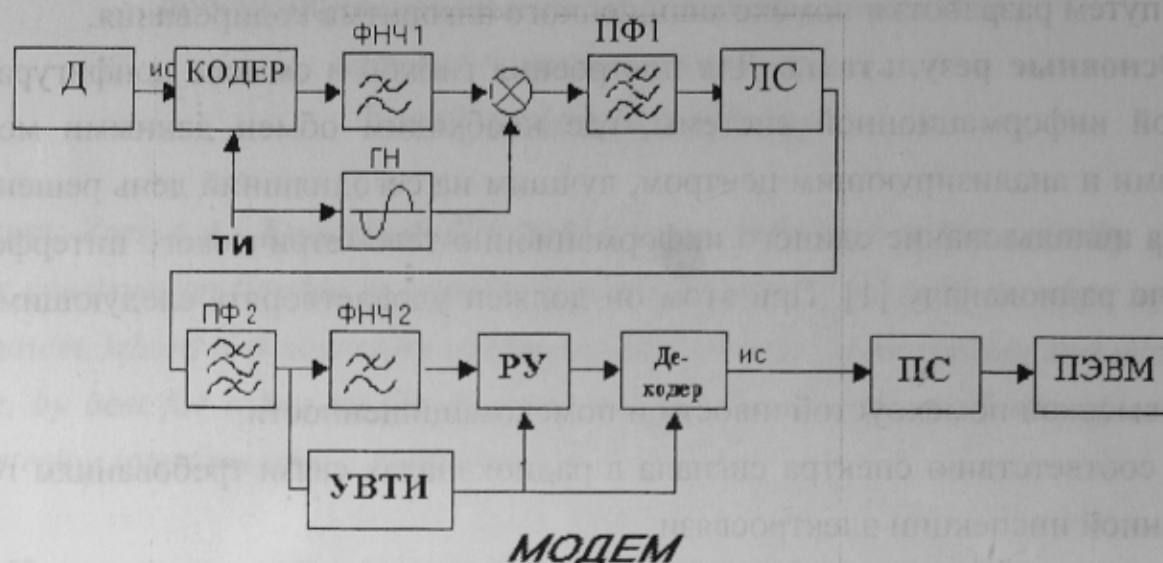
Рисунок 1 — Структурная схема информационно-телеметрического интерфейса системы
