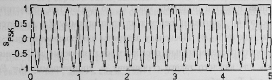
Рисунок 2 — Сигнал с 4-позиционной фазовой манипуляцией
