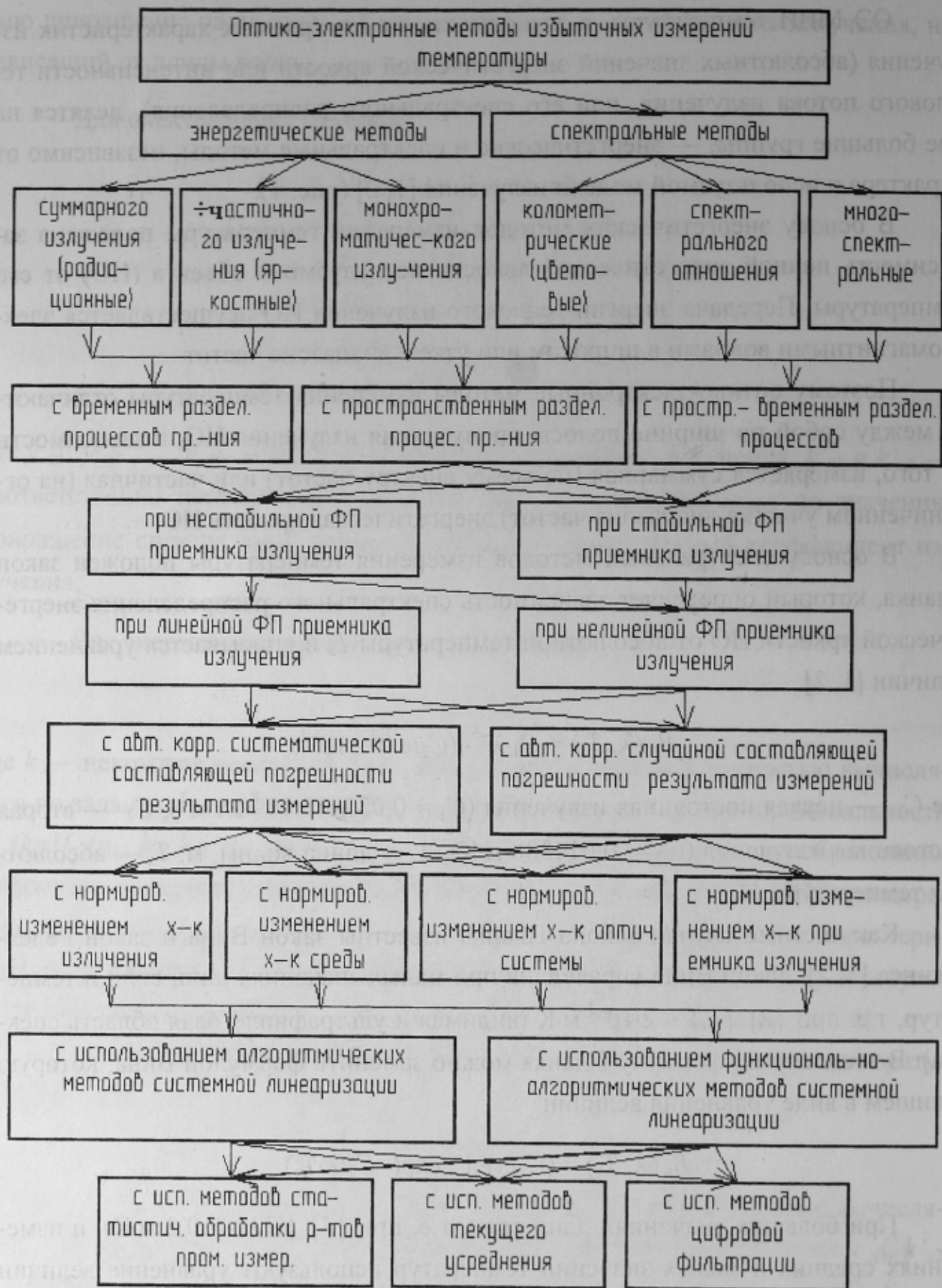
Рисунок 1 — Классификация оптико-электронных методов избыточных измерений температуры
