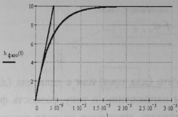
Рисунок 4 — Переходная характеристика канала измерения фаз
