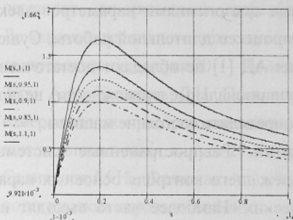
Рисунок 1 — Механическая характеристика при отклонениях напряжения сети
