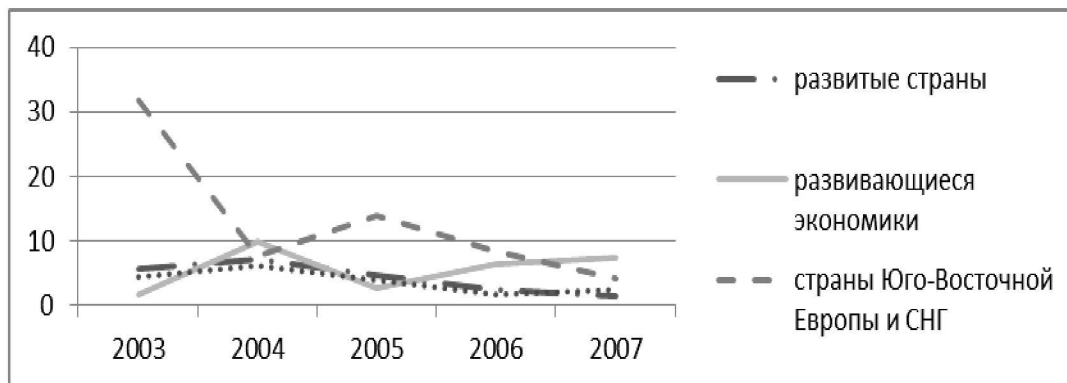
Рис. 1 Изменения коэффициентов структурных сдвигов по годам в разрезе исследуемых групп.
