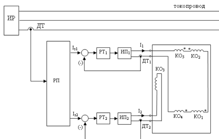
Рисунок 3 – Схема макета системы активного экранирования магнитного поля
