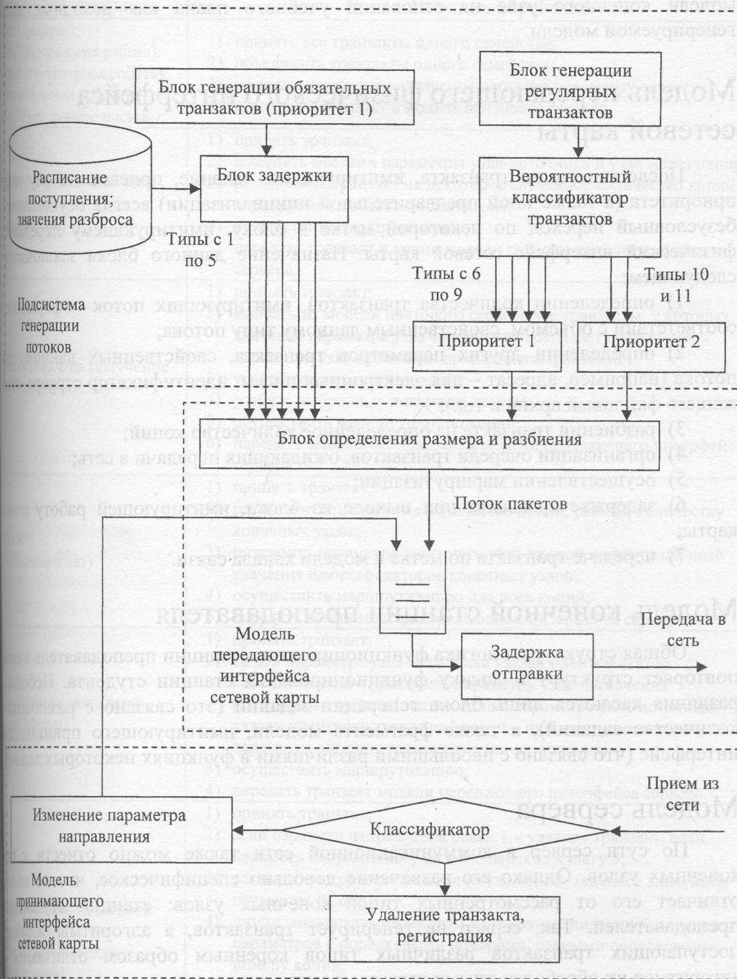
Рисунок 1 – Обобщенная схема функционирования модели станции студента
