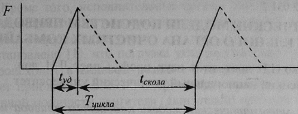
Рисунок 3 – Зависимость силы удара гидроимпульсной струи от времени
