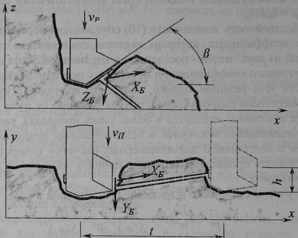
Рисунок 2 - Схема разрушения пласта резцом с рабочей боковой гранью
