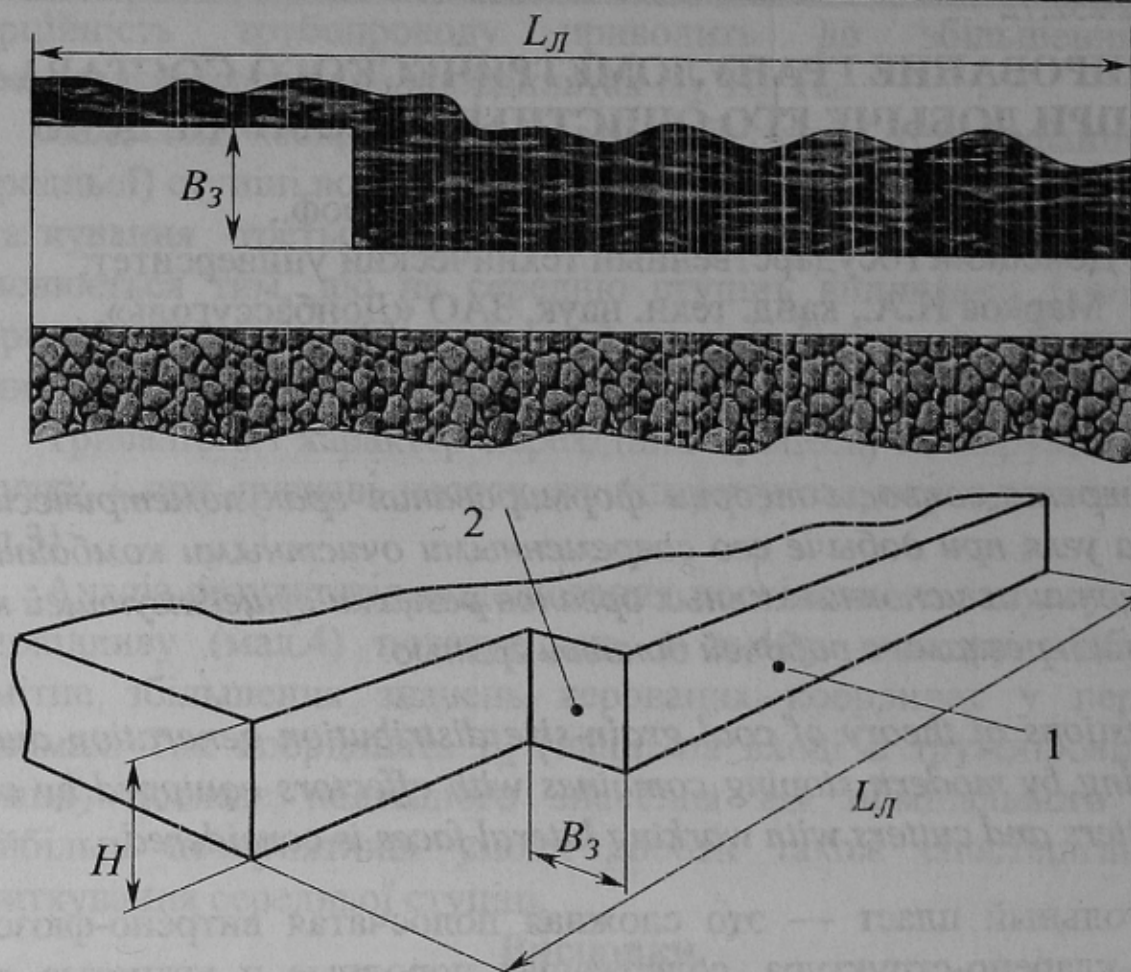
Рисунок 1. — Схема отработки пласта очистным комбайном
