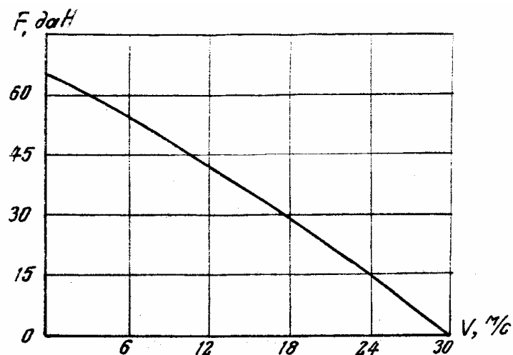
Рис. 3. Тяговая характеристика ЛИД с \tau=300 мм и ферромагнитным ротором
