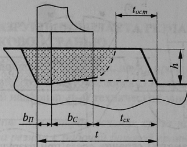
Рисунок 2 — Схема определения ширины остатка целика
