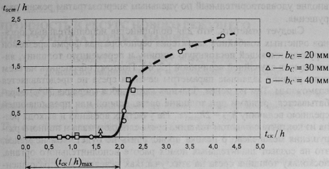
Рисунок 3 — Графік залежності ширини остатка целика от ширины свободно скальвающейся части целика, нормированных по толщине стружки
