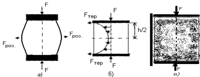
Рис. 1. Схеми стискування зразків:
