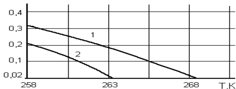
Рис. 2. Графіки залежності температури газогідрату від пористості для прояву ефекту самоконсервації при температурі повітря 273 К (крива 1) та 278 К (крива 2)
