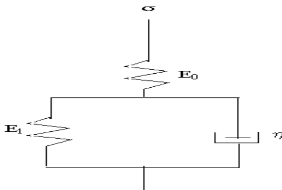
Рис. 8. Реологічна модель узагальненого пружно-в'язкого тіла (нормальна реологічна модель)
