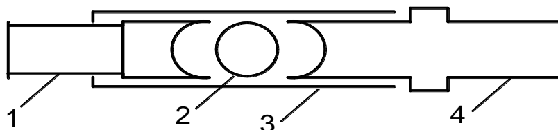
Рис. 3. Штмп для виготовлення газогідратних гранул: 1, 4 – верхній і нижній шток із півсферичними заглибинами; 2 – гранула газогідрату; 3 – корпус
