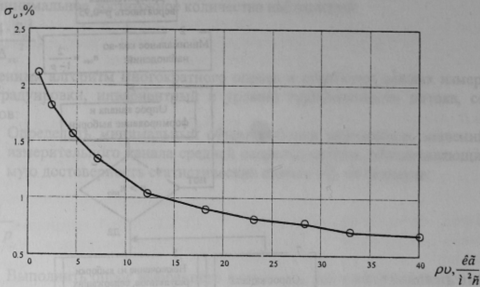
Рис.2. Зависимость уровня турбулентности потока в АС от средней скорости
