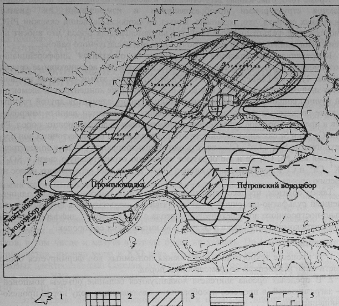
Рис. 1. Гидрохимическая зональность эпигенетического ореола: 1 — контур ореола суммарного загрязнения; 2 — хлоридно-сульфатные натриевые воды; 3 — сульфатно-хлоридные натрий-кальциевые воды; 4 — хлоридные кальциевые воды; 5 — гидрокарбонатно-хлоридные магний-кальциевые воды
