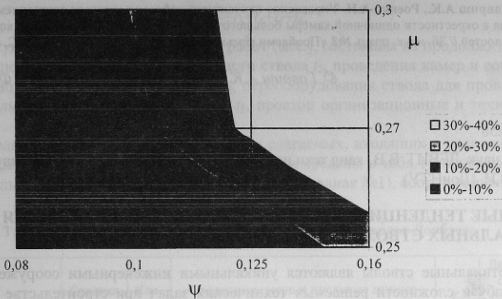
Рис. 3 Зависимость коэффициента \Delta K от физико-механических свойств пильных известняков
