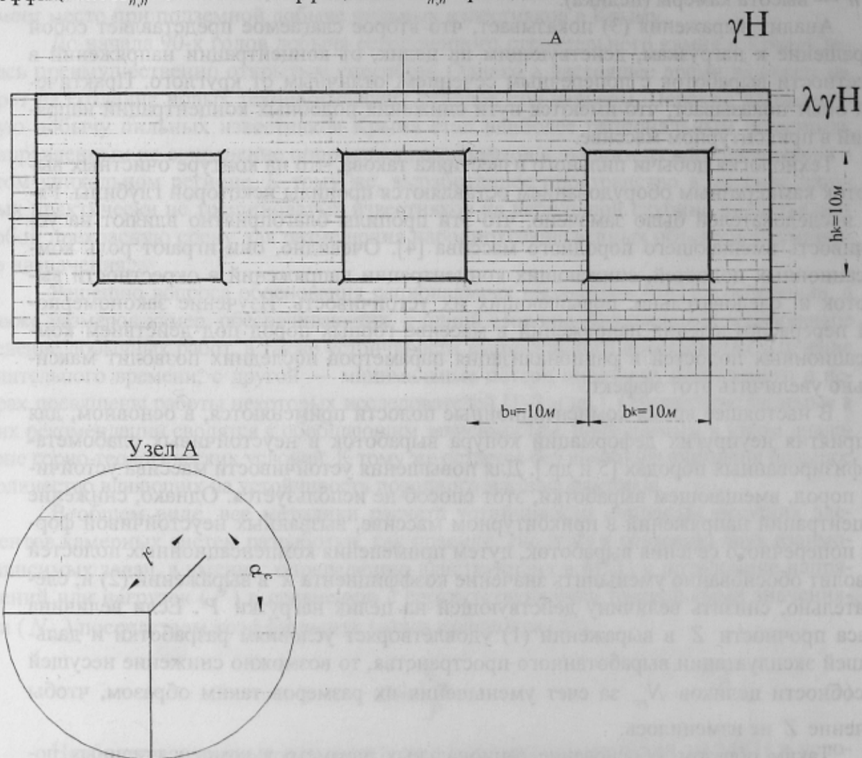
Рис. 1. Расчетная схема камерной системы разработки при исследовании влияния параметров компенсационных полостей на устойчивость подземных сооружений
