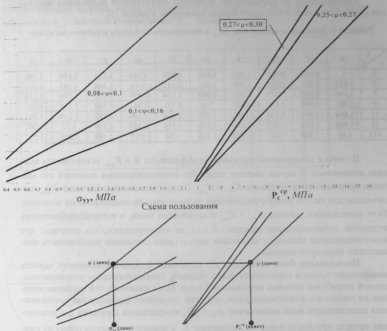
Рис. 2. Номограмма для определения средней величины внутреннего давления в пропилах P_c^{cp} в зависимости от вертикальной составляющей естественного поля напряжений
