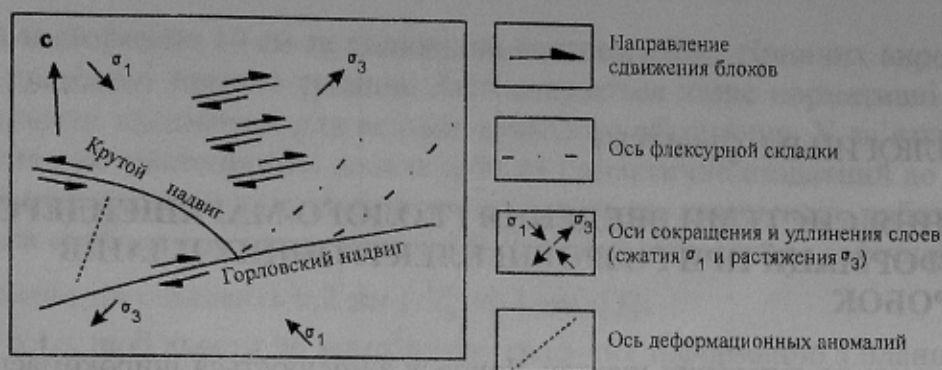
Рис.4. Схема формирования Горловского правого сдвиго-надвига
