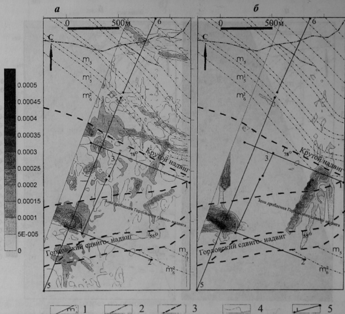
Рис. 3. Совмещенная геологическая карта участка исследований и карта модулей градиентов оседаний земной поверхности на период второй и третьей серии наблюдений: (а) с 1997 по 1999 гг.; (б) с 1999 по 2001 гг.: 1 — угольные пласты; 2 — тальвег овражно-балочной сети; 3 — тектонические нарушения; 4 — изолинии модулей градиентов оседаний земной поверхности; 5 — профильные линии геодезических наблюдений
