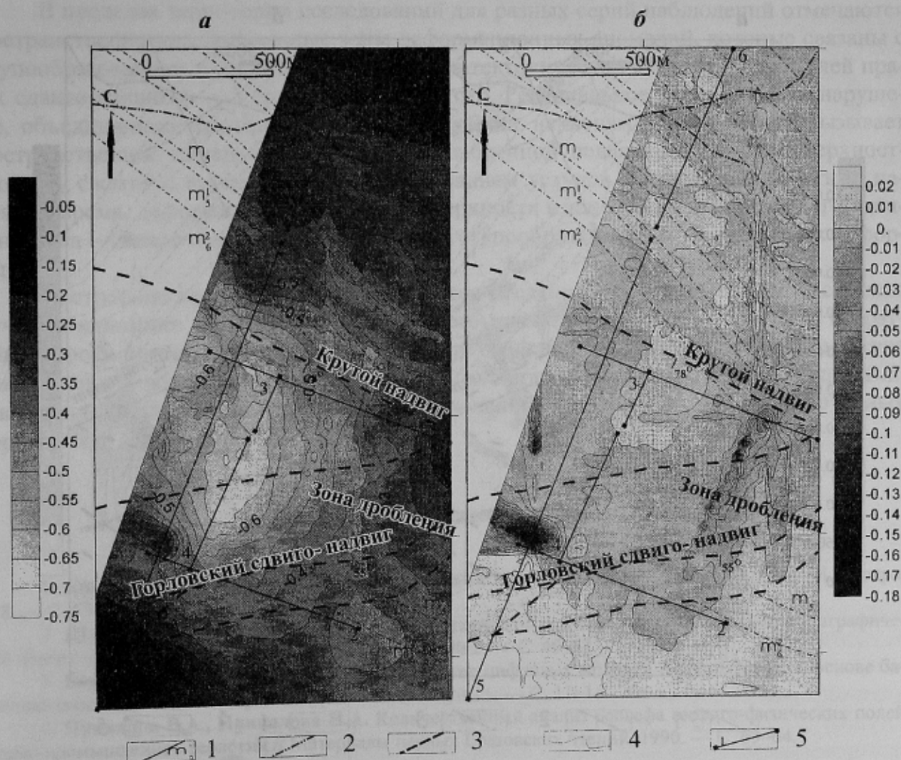
Рис. 2. Совмещенная геологическая карта участка исследований и карта оседаний земной поверхности на период второй и третьей серии наблюдений: (а) с 1997 по 1999 гг.; (б) с 1999 по 2001 гг.: 1 — угольные пласты; 2 — тальвег овражно-балочной сети; 3 — тектонические нарушения; 4 — изолинии оседаний земной поверхности; 5 — профильные линии геодезических наблюдений
