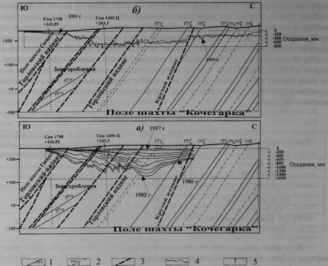
Рис. 1. Геологический разрез по основным и фланговым квершлагам, совмещенный с графиками оседания земной поверхности: а) на период серий наблюдений в эксплуатационный период шахты «Кочегарка»; б) на период серий наблюдений после консервации: 1 — угольные пласты рабочей мощности; 2 — угольные пласты нерабочей мощности; 3 — тектонические нарушения; 4 — кривая оседаний земной поверхности; 5 — разведочные скважины
