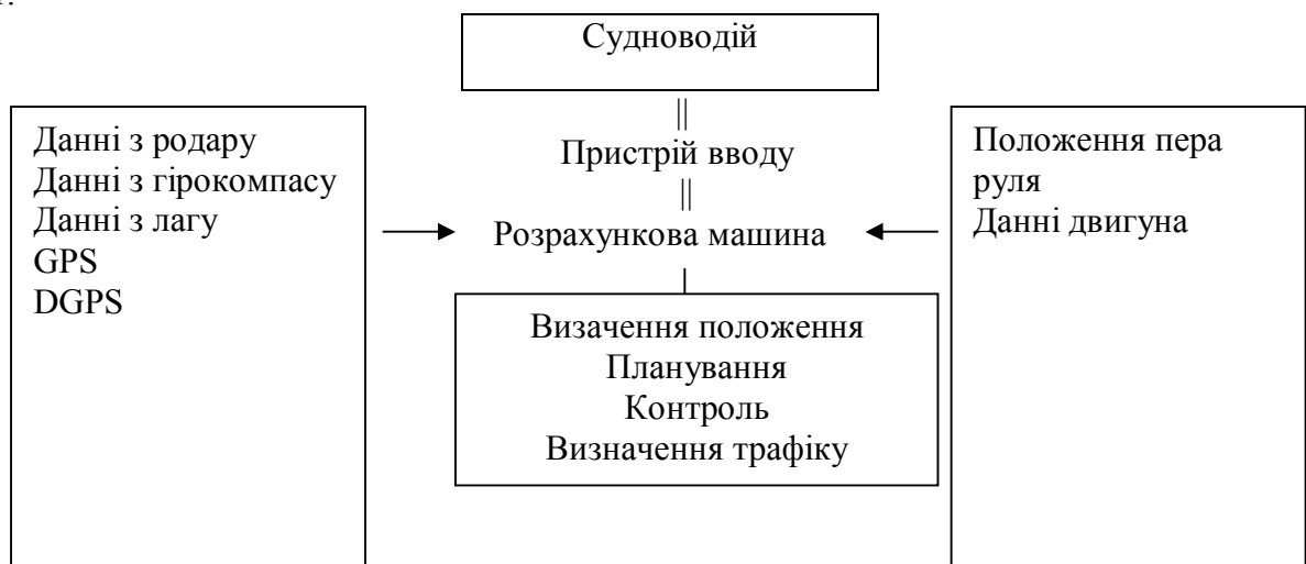
Рисунок 1 – Схема навігаційної інтегрованої системи(тренажеру)
