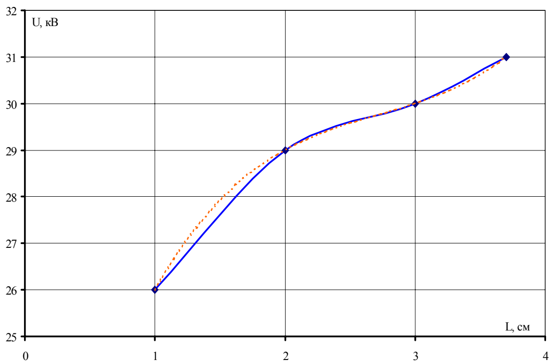
Рисунок 3 - Зависимость напряжения гашения от расстояния между правым электродом и основанием источника пламени
