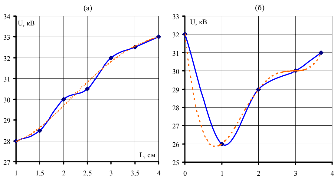
Рисунок 2 - Зависимость напряжения гашения от расстояния между правым электродом и основанием источника пламени
