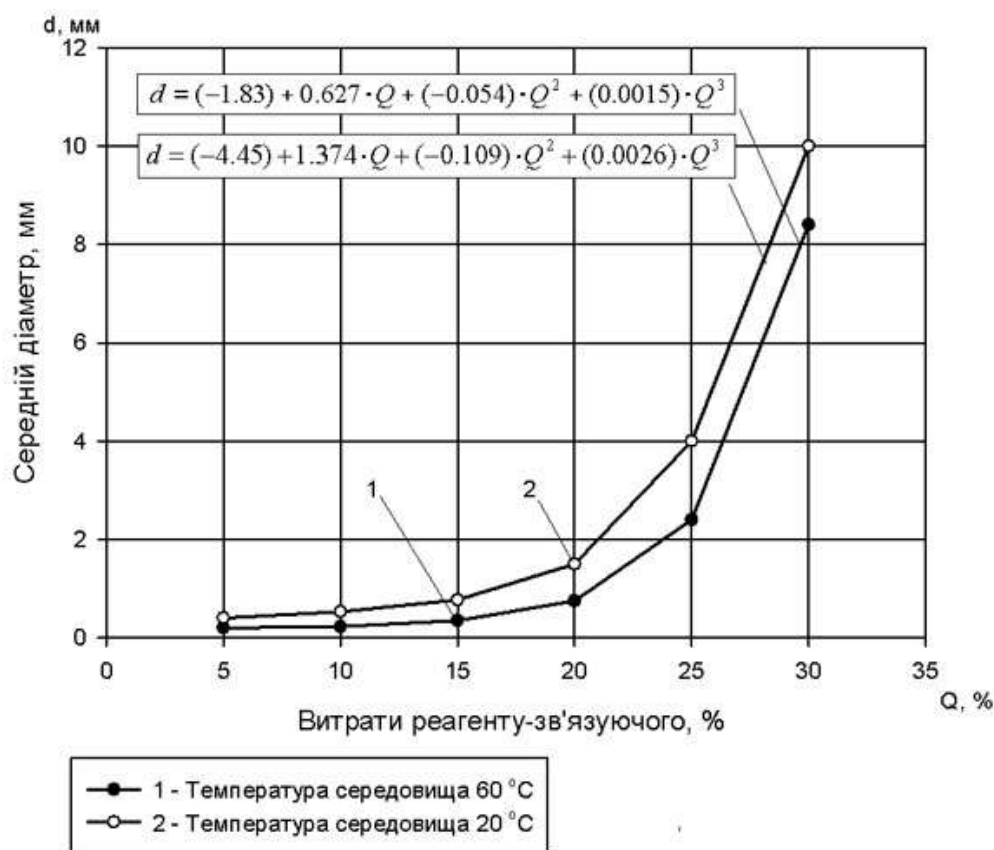
Рис.1 - Залежності середньої крупності гранул від витрат реагента-зв'язуючого для різної температури середовища пелетування
