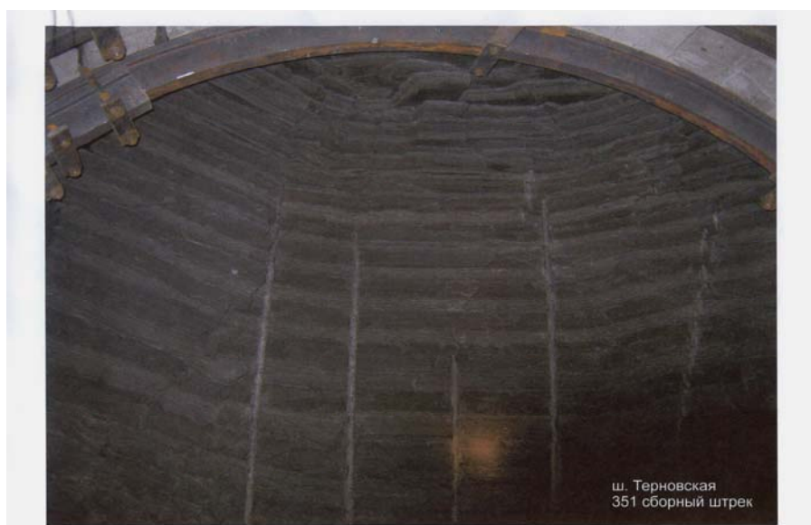
Рис.10 Состояние пород кровли в месте перекрепления 351 сборного штрека шахты Тернопольская.
