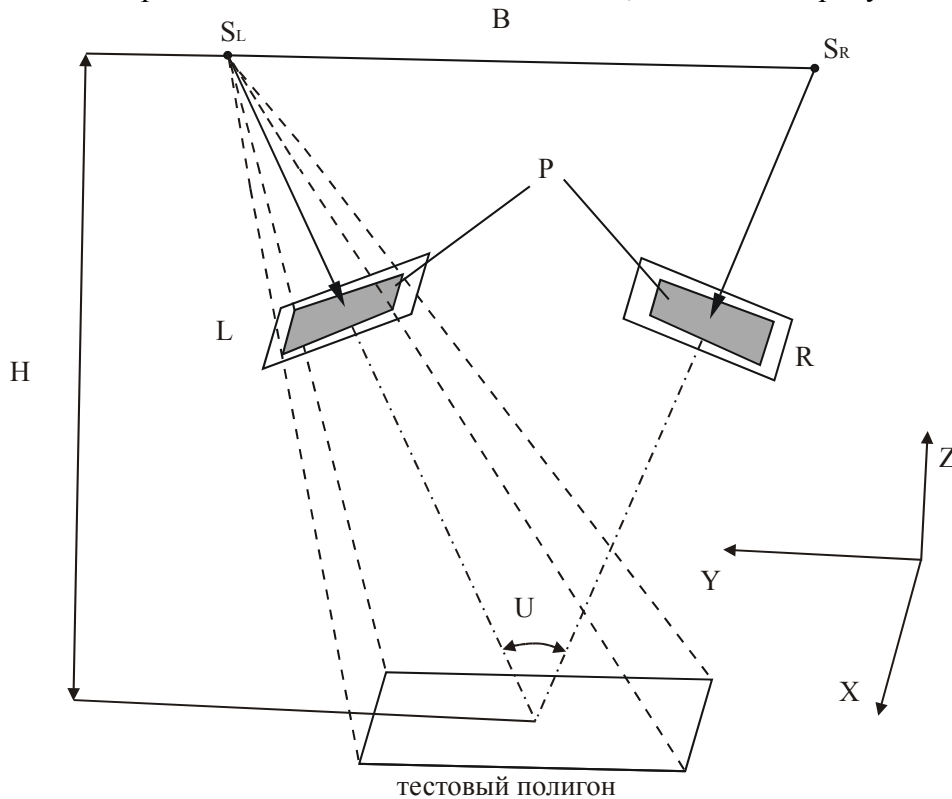
Рис. 1. Параметры фотографирования
