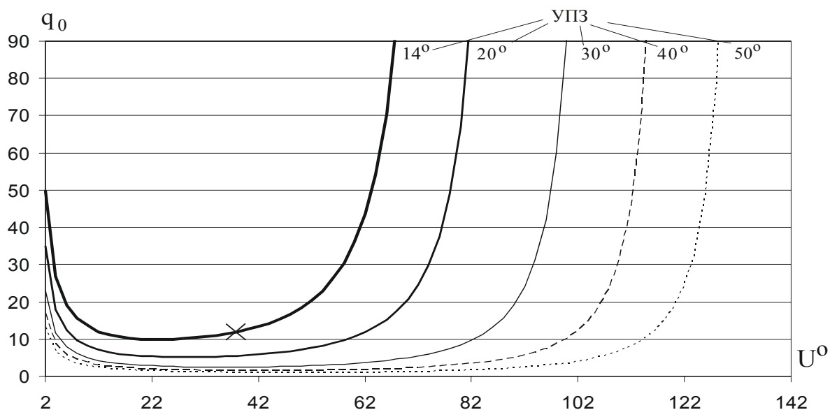
Рис. 3. Точность определения координат главной точки снимка в зависимости от угла конвергенции стереопар
