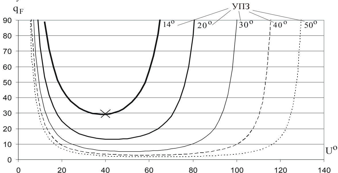
Рис. 2. Точность определения фокусного расстояния камер в зависимости от угла конвергенции стереопар
