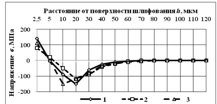
Рис. 1. Зависимость остаточных напряжений от способа шлифования титанового сплава VT14 кругами AC6 100/80 (а), AC6 160/125 (б), AC6 250/200 (в): 1 – АЭШ; 2 – шлифование с электроэрозионной правкой в автономной зоне; 3 – алмазное шлифование
