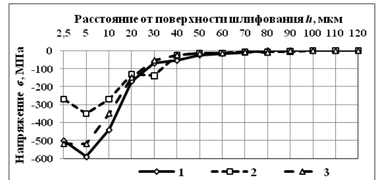
Рис. 2. Зависимость остаточных напряжений от способа шлифования быстрорежущей стали Р6М5Ф3 кругами AC6 100/80 (а), AC6 160/125 (б), AC6 250/200 (в): 1 – АЭЭШ; 2 – шлифование с электроэрозионной правкой в автономной зоне; 3 – алмазное шлифование
