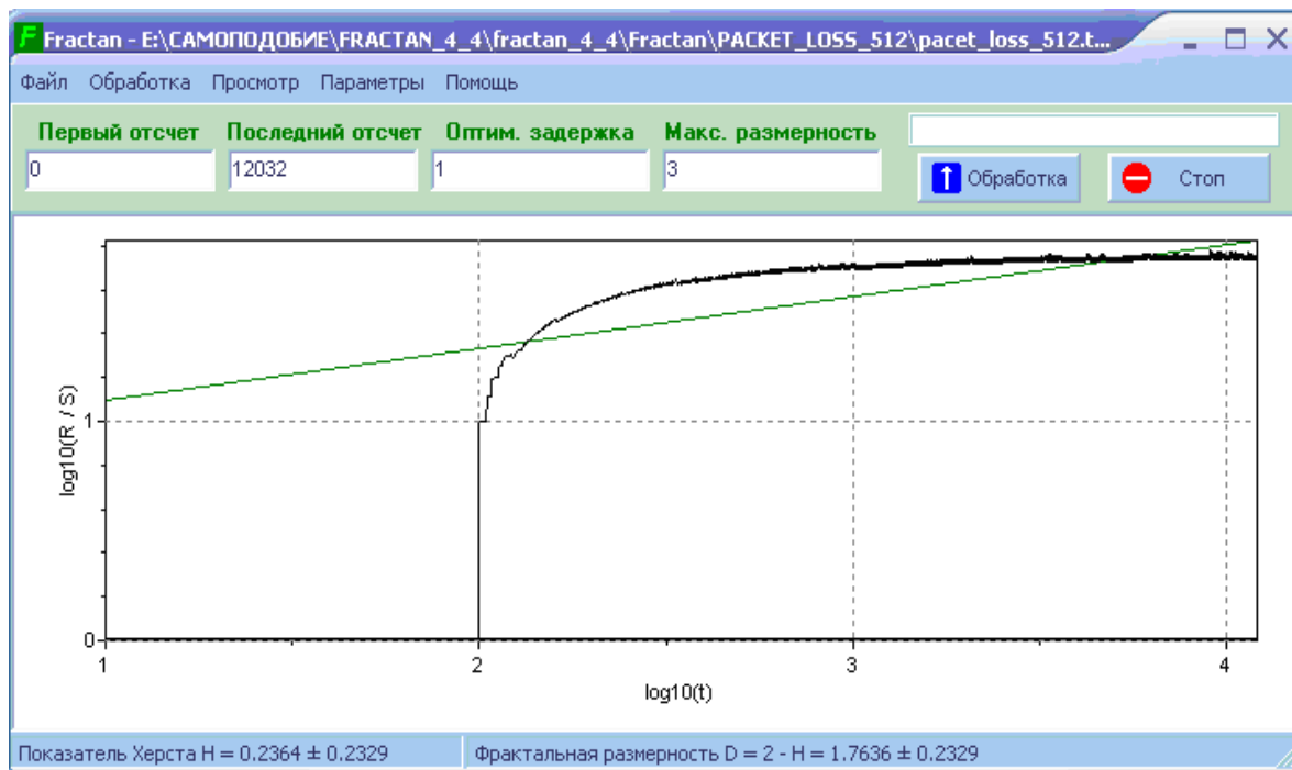
Рисунок 6.- Определение показателя Херста
