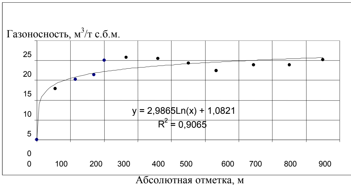
Рис.1. График изменения метаноносности угольных пластов с глубиной и повышением степени метаморфизма
