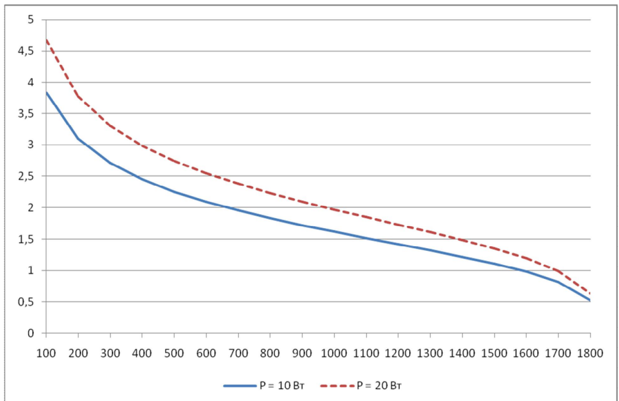
Рисунок 2.4 - Залежність радіусу сайту від пропускної здатності downstream каналу
