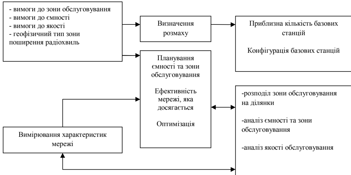
Рисунок 2.1 - Процес планування радіомережі 3G
