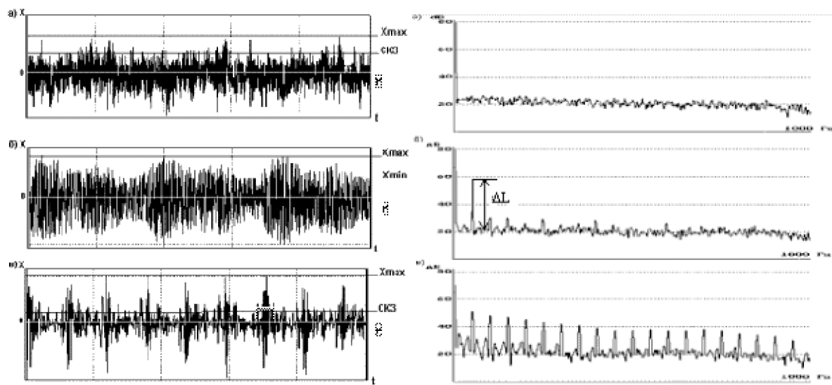
Рис. 3 - Временные сигналы высокочастотной вибрации подшипника качения и спектры ее огибающей:
