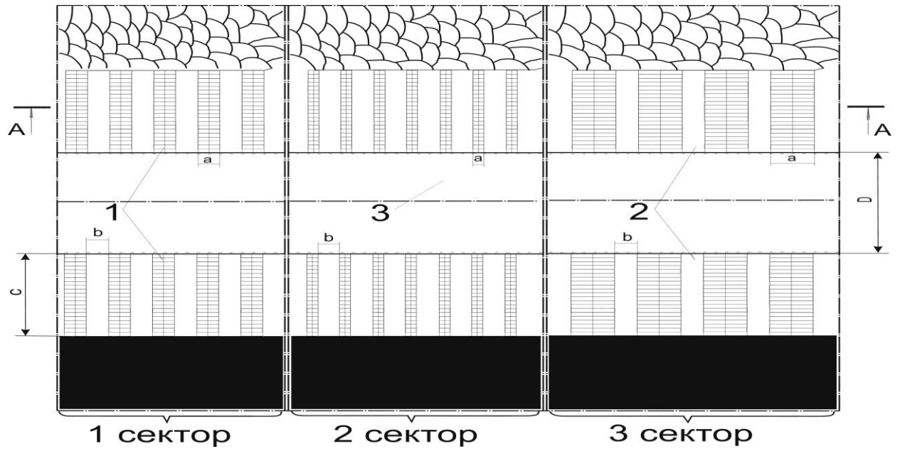
Рис.7. Схема расположения охранных сооружений (1) с компенсационными полостями (2) вдоль выработки (3) (где a – ширина охранных сооружений, b – ширина компенсационной полости между охранными сооружениями, D – ширина выработки, C – длина охранных сооружений).
