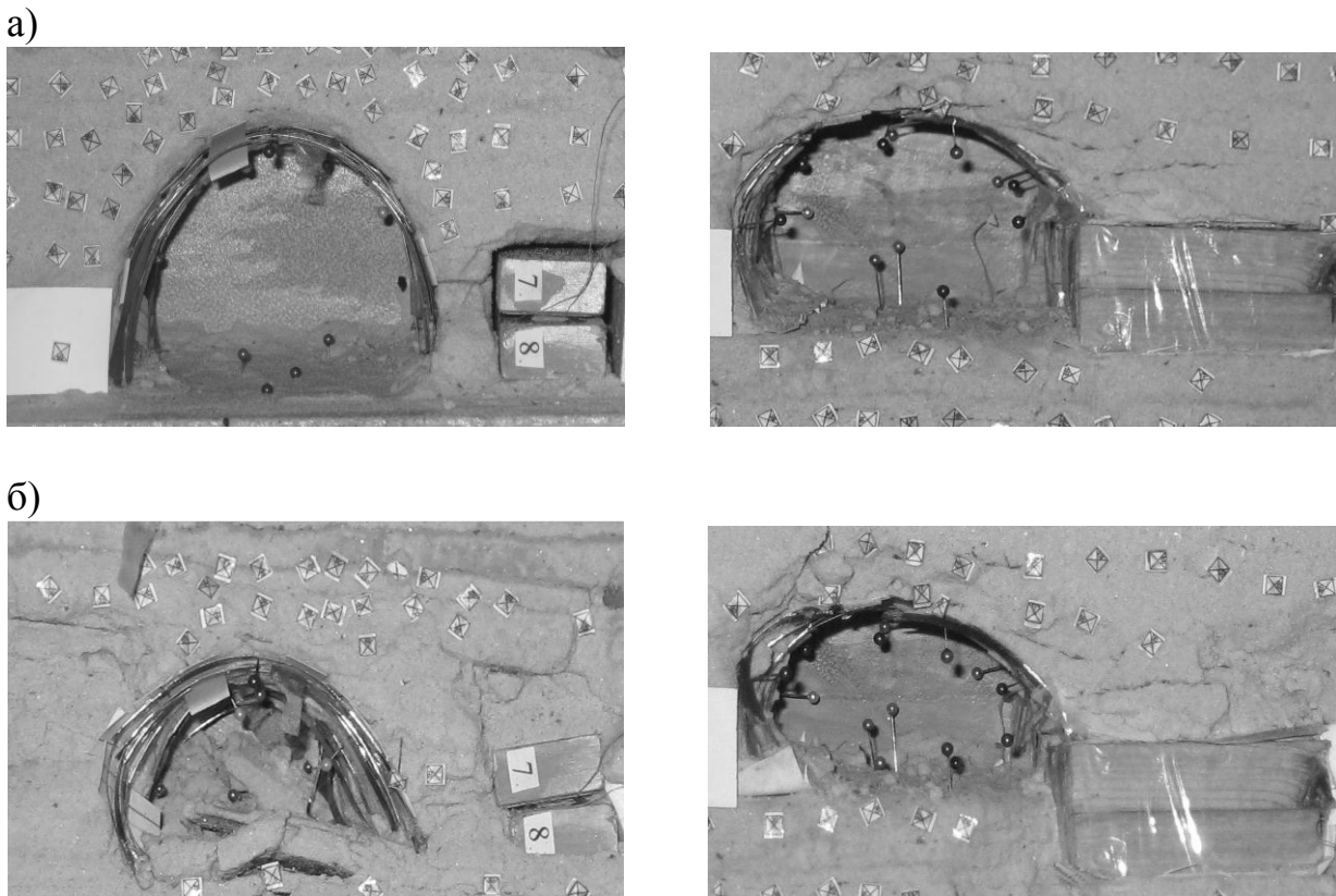
Рис.12. Общий вид выработок в моделях до (а) и после отработки (б) при традиционном (левая часть рисунка) и предлагаемом (правая часть рисунка) способах охраны.
