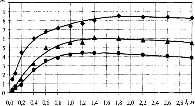
Рисунок 1 - Зависимости кинетической энергии импульсной струи от расстояния между насадком генератора и преградой
